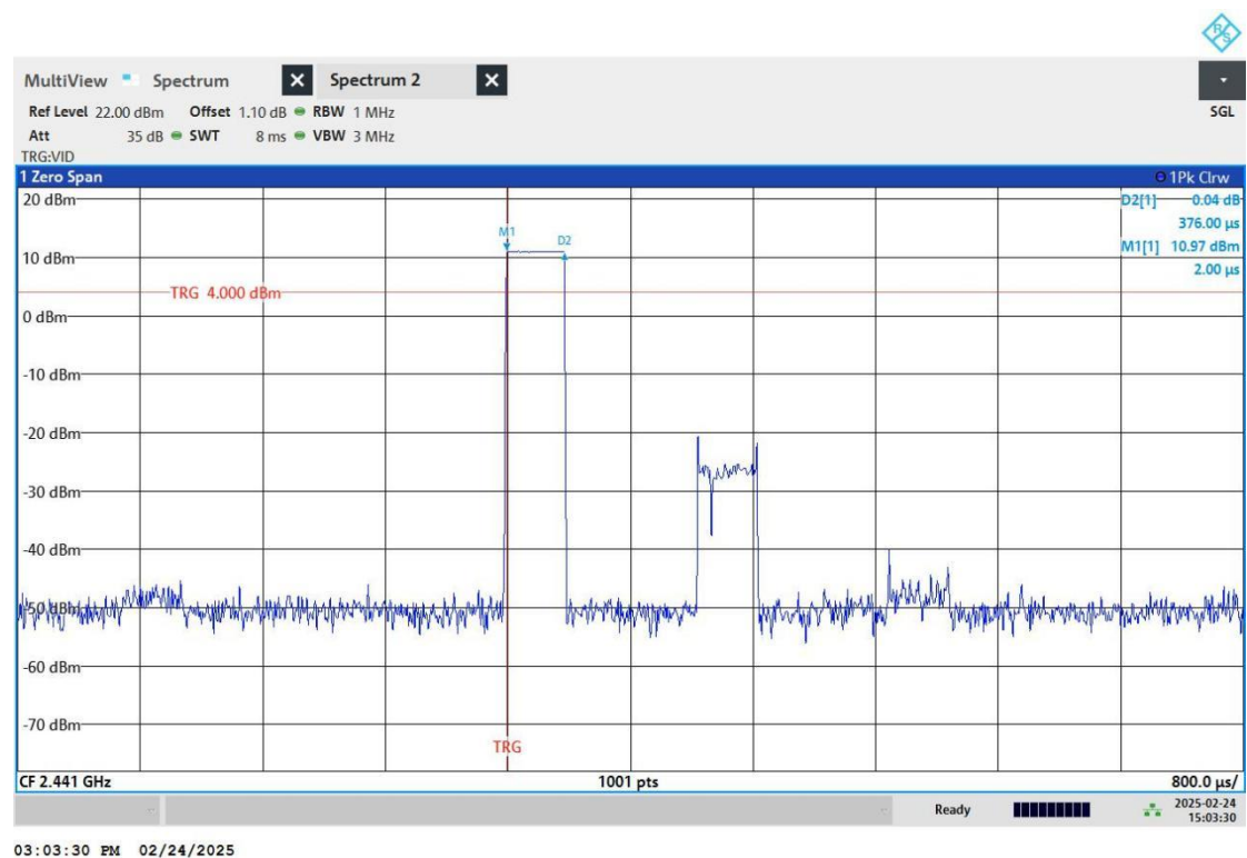
DH1_ANT7_Hop
