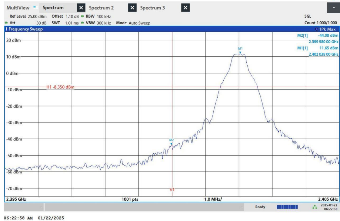
DH5_ANT7_Low_2402
