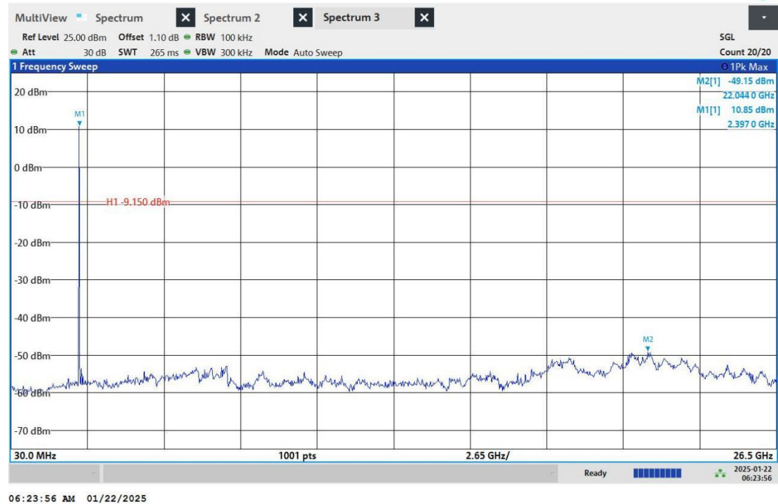
DH5_ANT7_2402_30~26500
