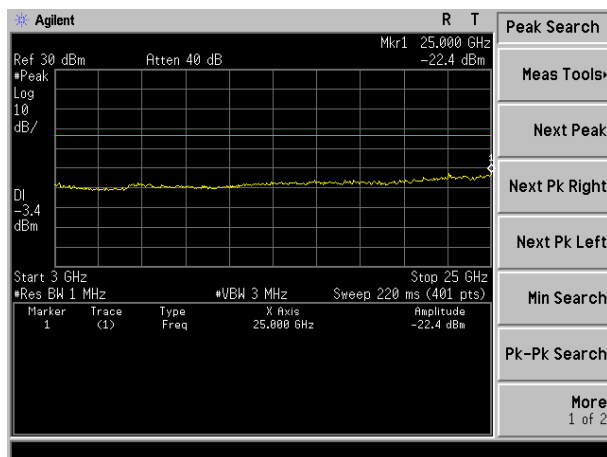
3GHz ~25GHz
