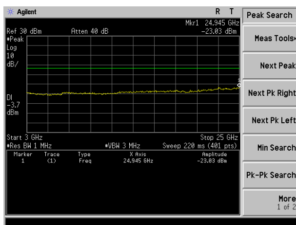
3GHz ~25GHz
