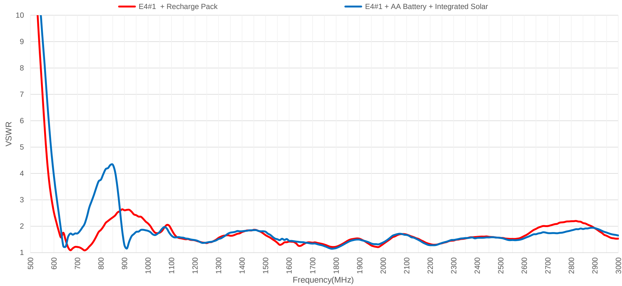
VSWR
