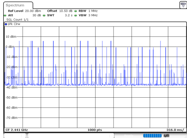
2DH5_Hopping
