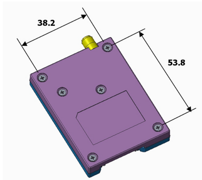
Fig 2. CM105, Bottom
