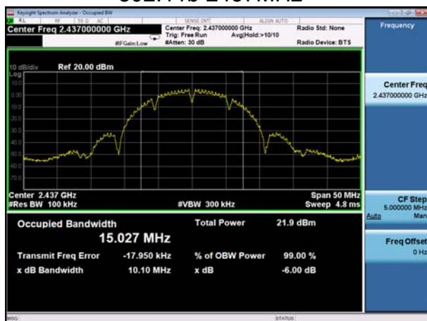
802.11b 2437MHz
