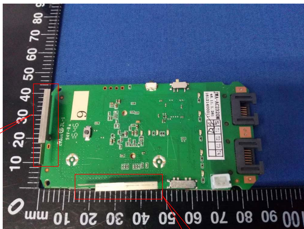
5G ANT 2
