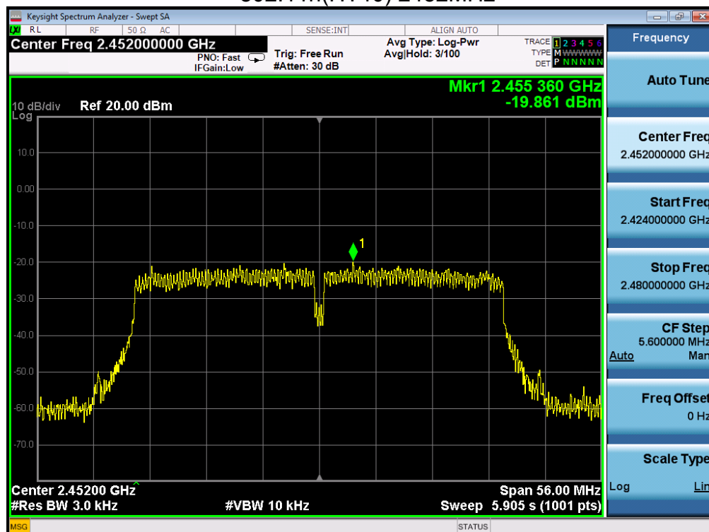
802.11n(HT40) 2452MHz
