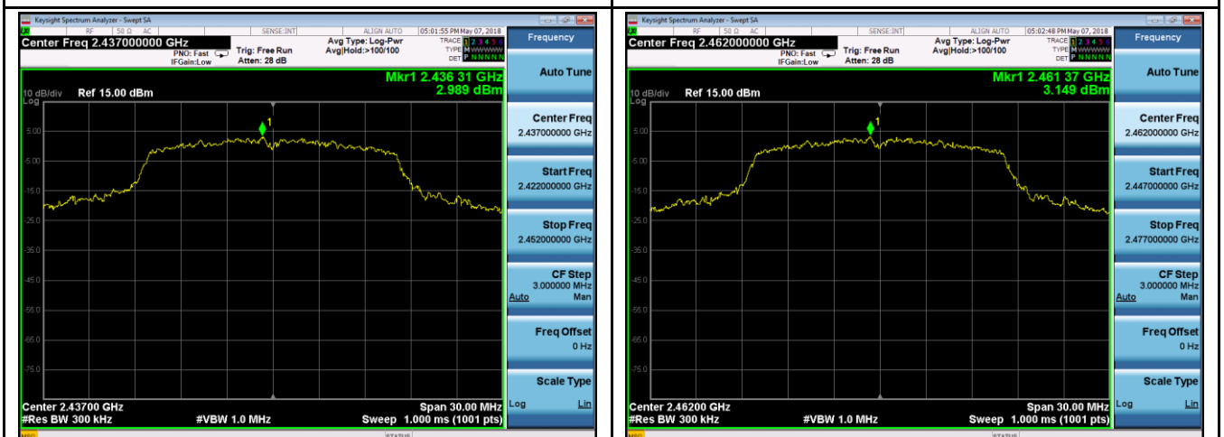
802.11g - AV Output power - Mid CH 2437
