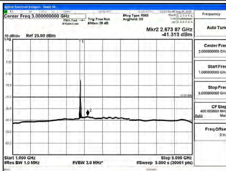
Band41-20MHz-QPSK-39750-1RB#0-Range4:1000~5000MHz
