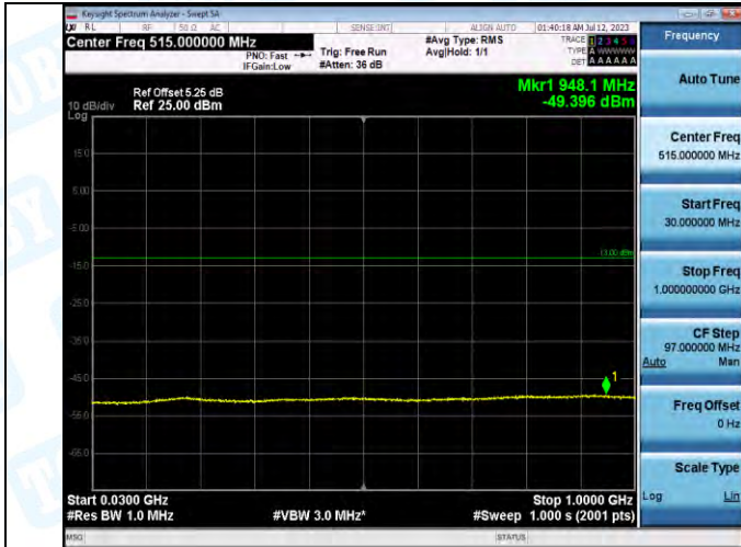
Band2-9400-1-30~1000MHz-PASS
