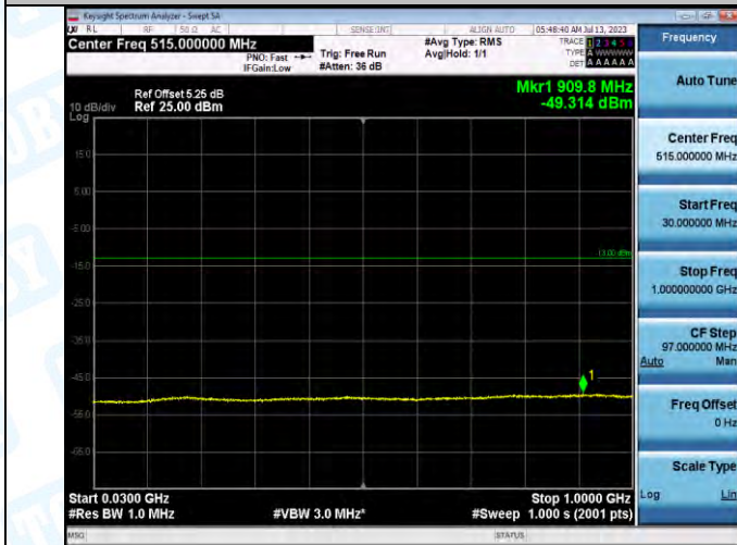
Band2-9538-5-30~1000MHz-PASS
