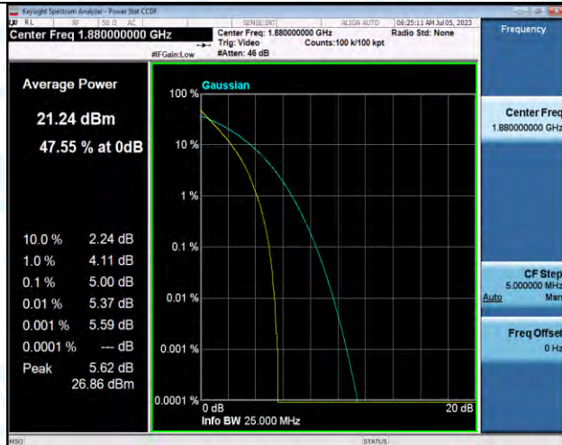
Band2-10MHz-QPSK-18900-50RB#0-PASS
