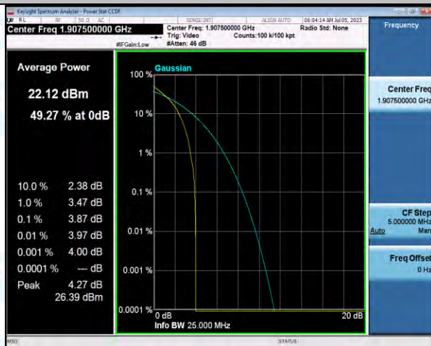
Band2-5MHz-QPSK-19175-1RB#0-PASS
