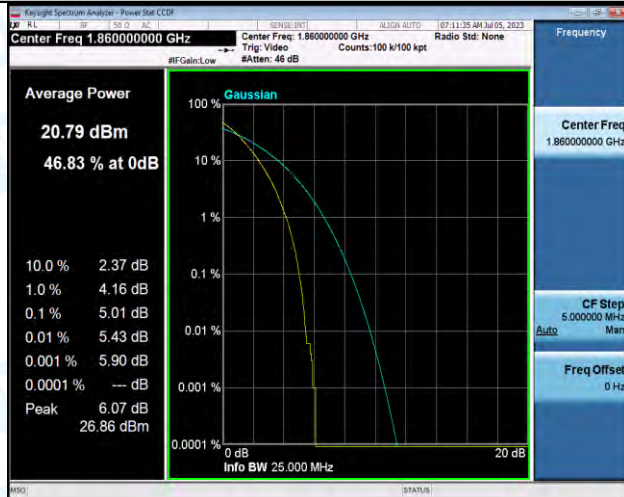
Band2-20MHz-QPSK-18700-100RB#0-PASS
