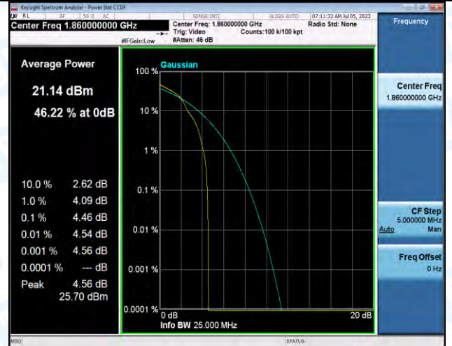
Band2-20MHz-16QAM-18700-1RB#0-PASS
