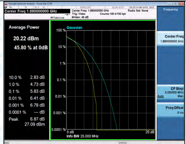
Band2-10MHz-16QAM-18900-50RB#0-PASS
