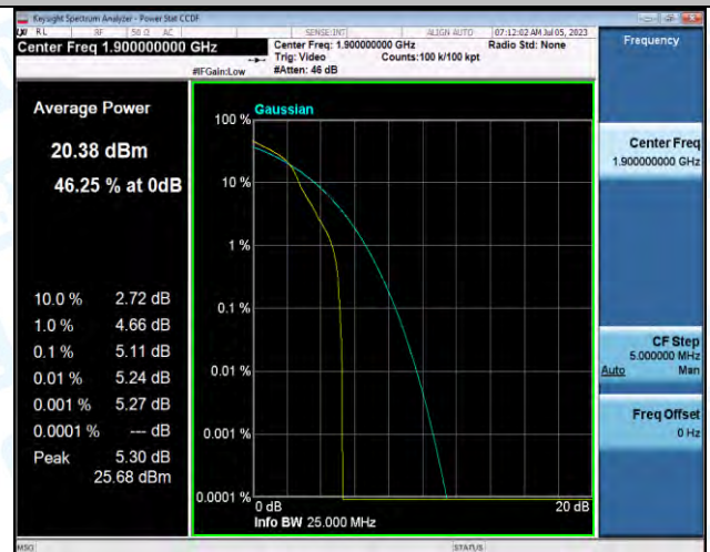
Band2-20MHz-16QAM-19100-1RB#0-PASS
