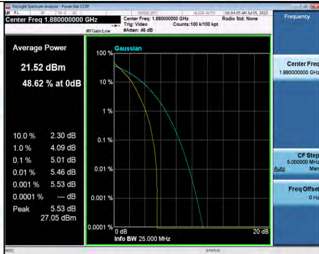
Band2-5MHz-QPSK-18900-25RB#0-PASS
