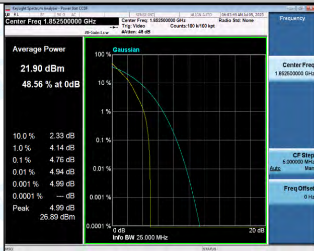
Band2-5MHz-QPSK-18625-25RB#0-PASS
