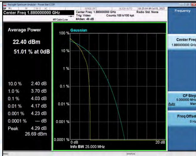
Band2-10MHz-QPSK-18900-1RB#0-PASS
