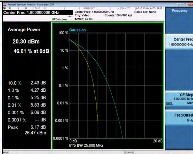
Band2-20MHz-QPSK-19100-100RB#0-PASS
