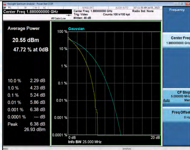
Band2-20MHz-QPSK-18900-100RB#0-PASS
