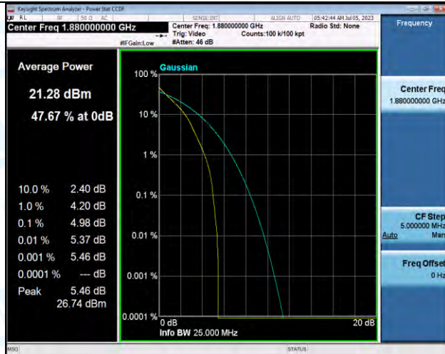
Band2-3MHz-QPSK-18900-15RB#0-PASS
