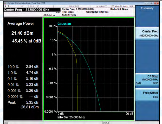
Band2-5MHz-16QAM-18625-1RB#0-PASS
