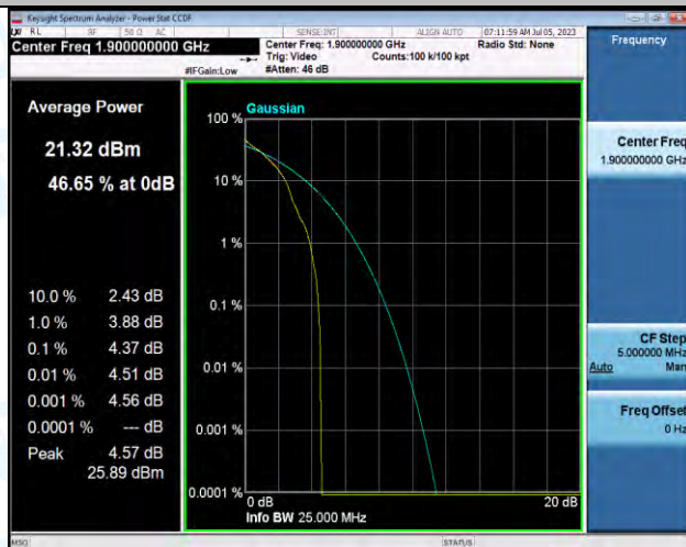
Band2-20MHz-QPSK-19100-1RB#0-PASS
