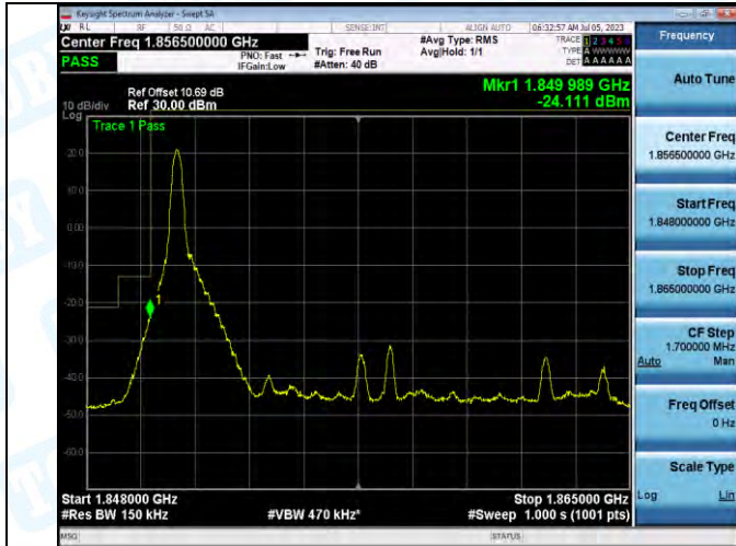
Band2_Band2_15MHz_QPSK_18675_1RB#0
