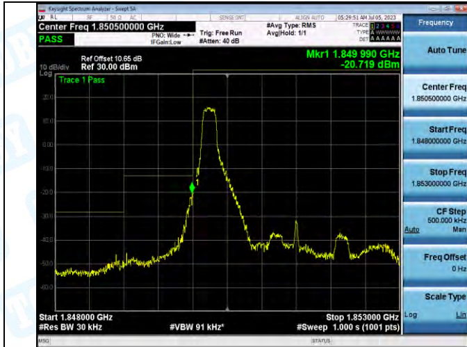
Band2_Band2_3MHz_QPSK_18615_1RB#0
