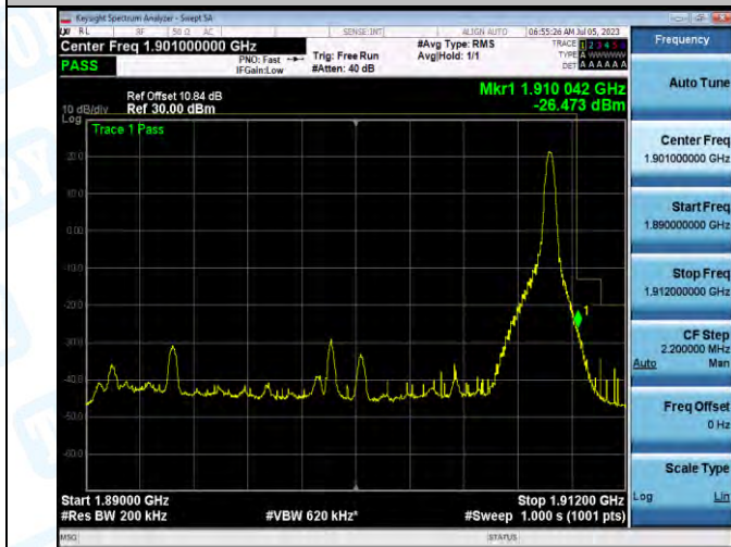
Band2_Band2_20MHz_QPSK_19100_1RB#99
