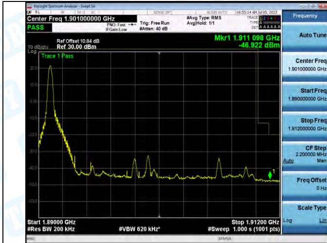
Band2_Band2_20MHz_QPSK_19100_1RB#0
