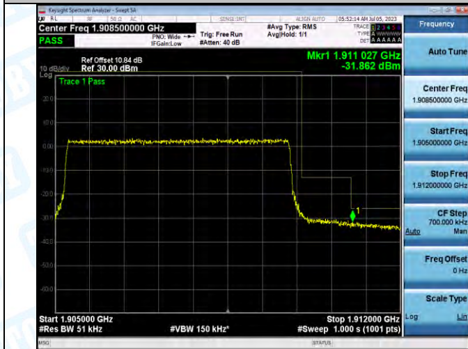
Band2_Band2_5MHz_QPSK_19175_25RB#0
