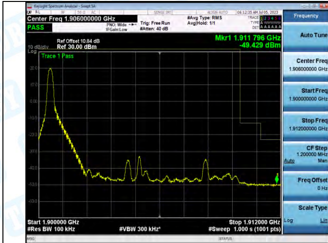
Band2_Band2_10MHz_QPSK_19150_1RB#0
