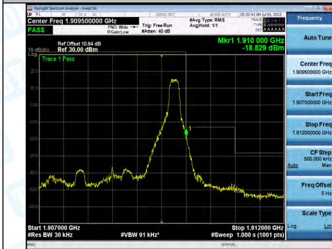
Band2_Band2_3MHz_QPSK_19185_1RB#14
