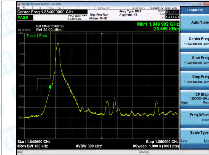
Band2_Band2_10MHz_QPSK_18650_1RB#0
