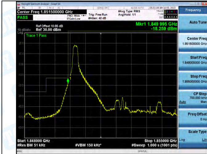
Band2_Band2_5MHz_QPSK_18625_1RB#0
