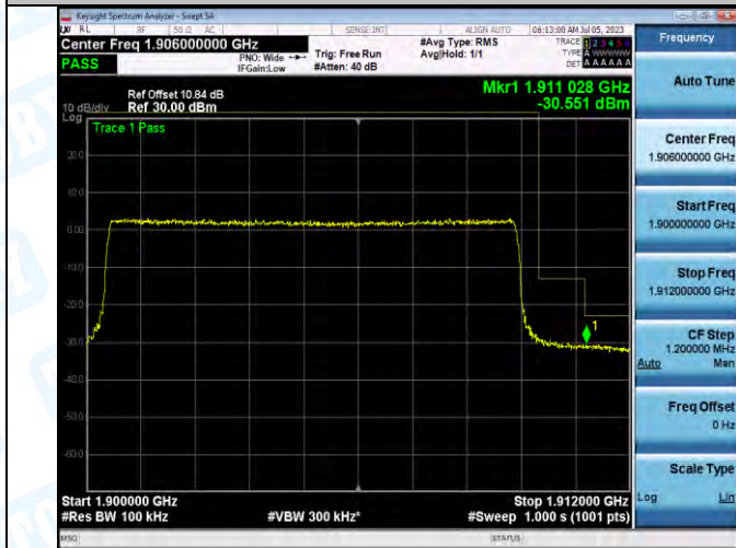
Band2_Band2_10MHz_QPSK_19150_50RB#0
