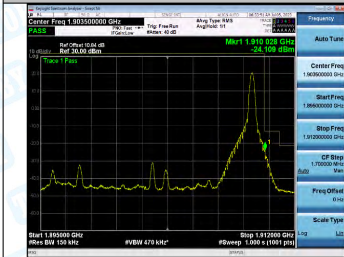
Band2_Band2_15MHz_QPSK_19125_1RB#74
