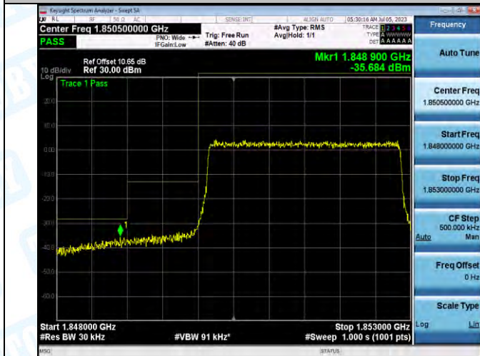
Band2_Band2_3MHz_QPSK_18615_15RB#0
