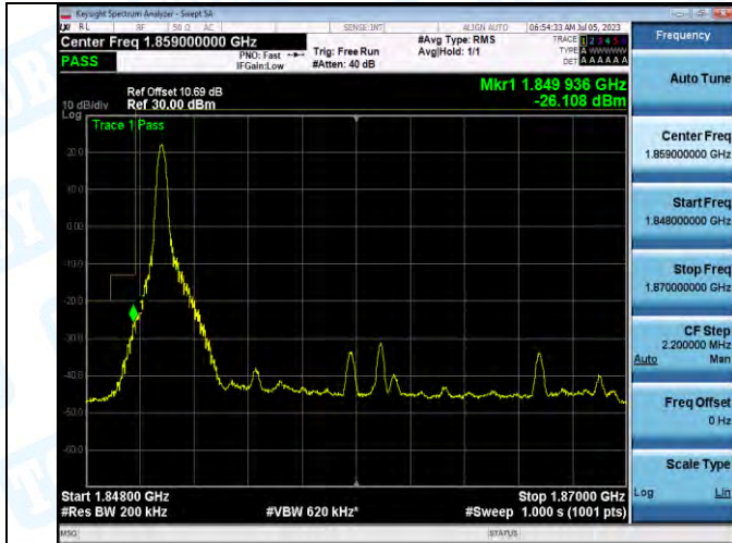
Band2_Band2_20MHz_QPSK_18700_1RB#0
