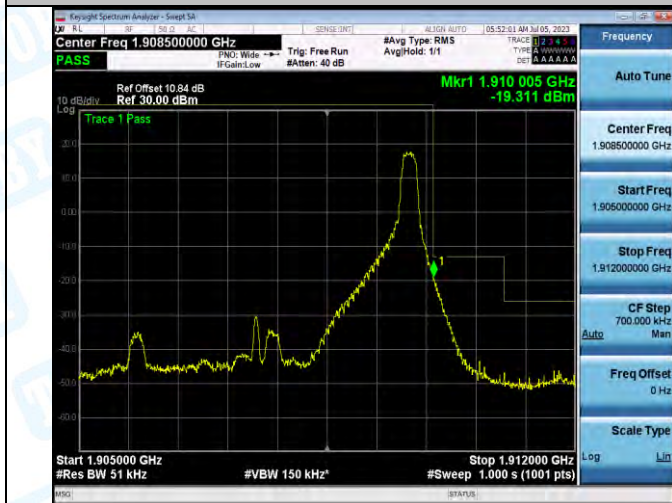
Band2_Band2_5MHz_QPSK_19175_1RB#24
