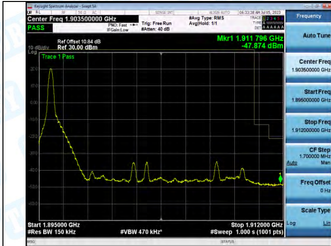
Band2_Band2_15MHz_QPSK_19125_1RB#0
