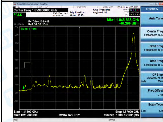
Band2_Band2_20MHz_QPSK_18700_1RB#99
