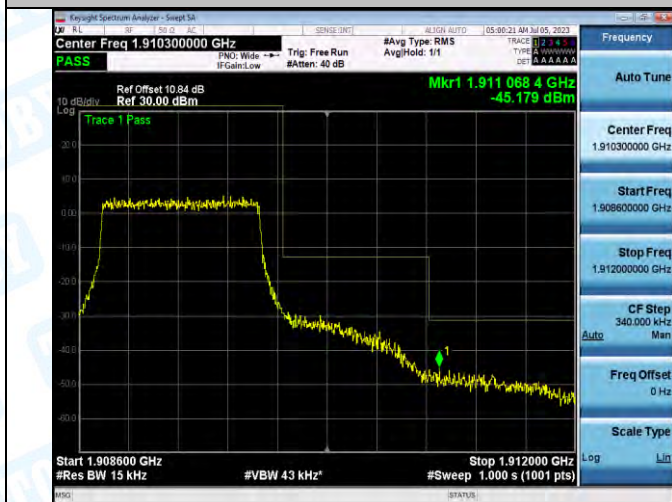
Band2_Band2_1.4MHz_QPSK_19193_6RB#0
