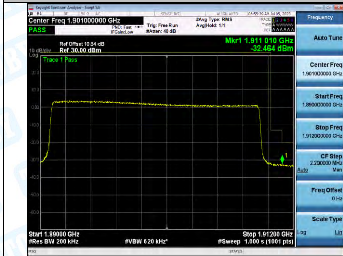
Band2_Band2_20MHz_QPSK_19100_100RB#0
