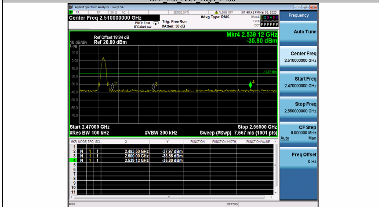
BLE 2M Ant1 High 2480
