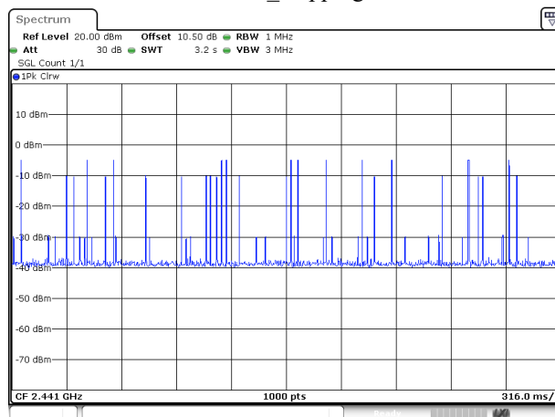
2DH5_Hopping
