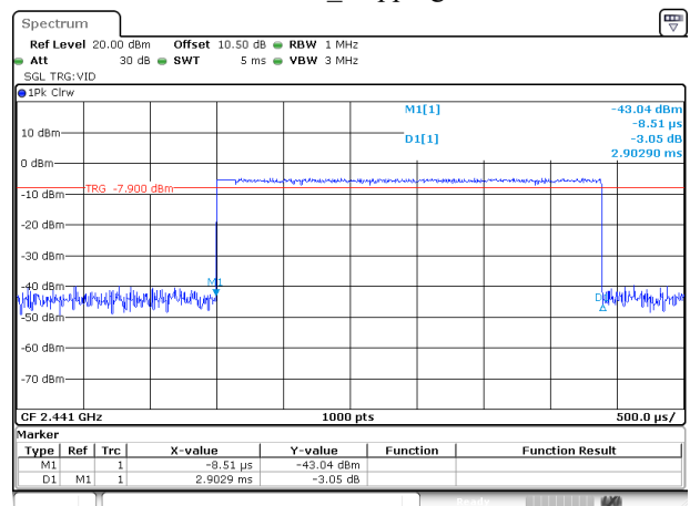
2DH5_Hopping
