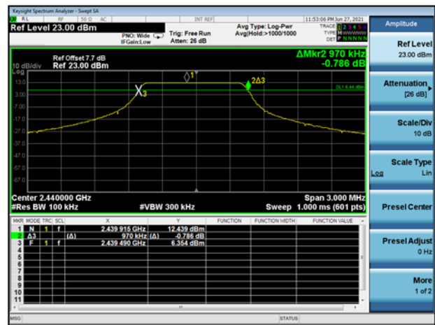
LoRa(812kHz) MIDDLE CHANNEL
