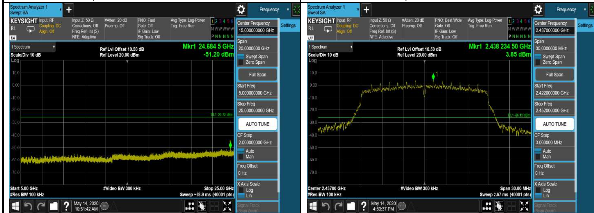
802.11n(HT20),2437MHz,Ant1,Plot 2,Band Edge
