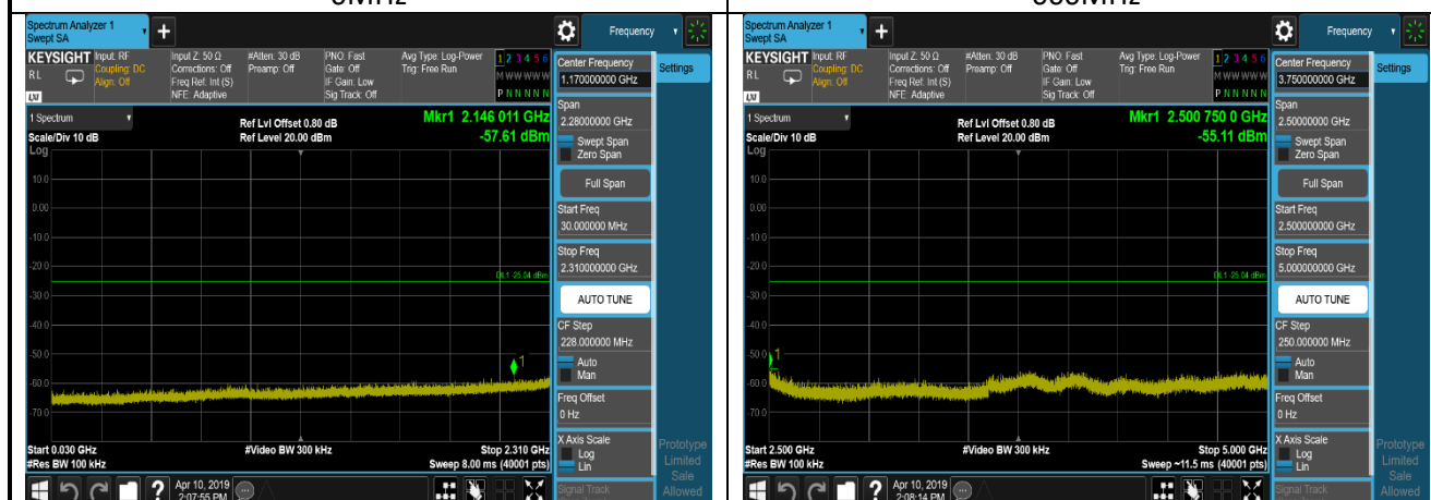
802.11g,2462MHz,Ant0,Plot 5,5000MHz~2500MHz
