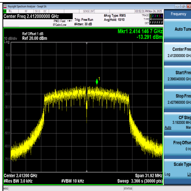
11N20ISO-Ant1-2412-PASS
