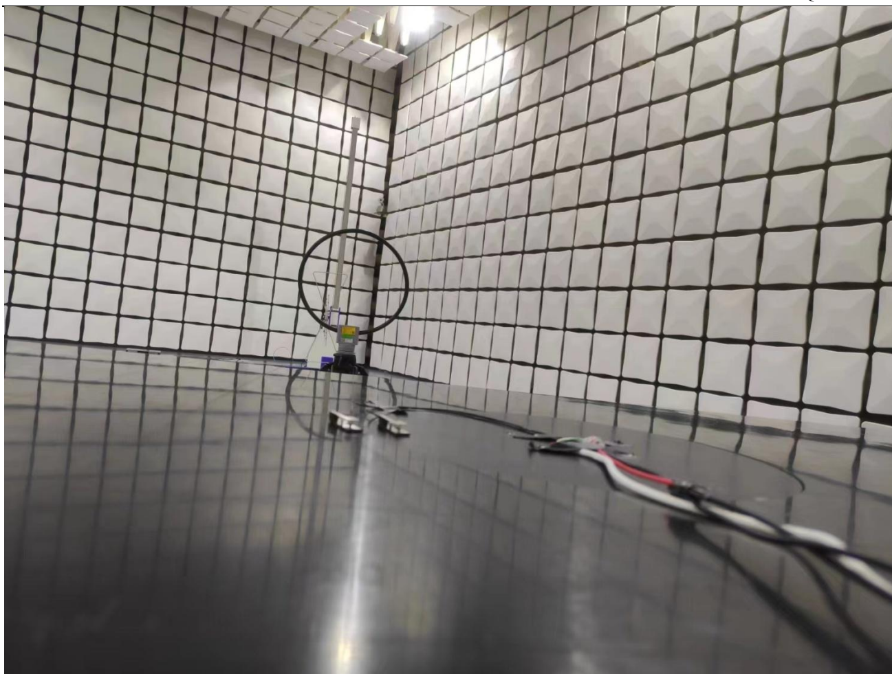
RE9KHz~30MHz
