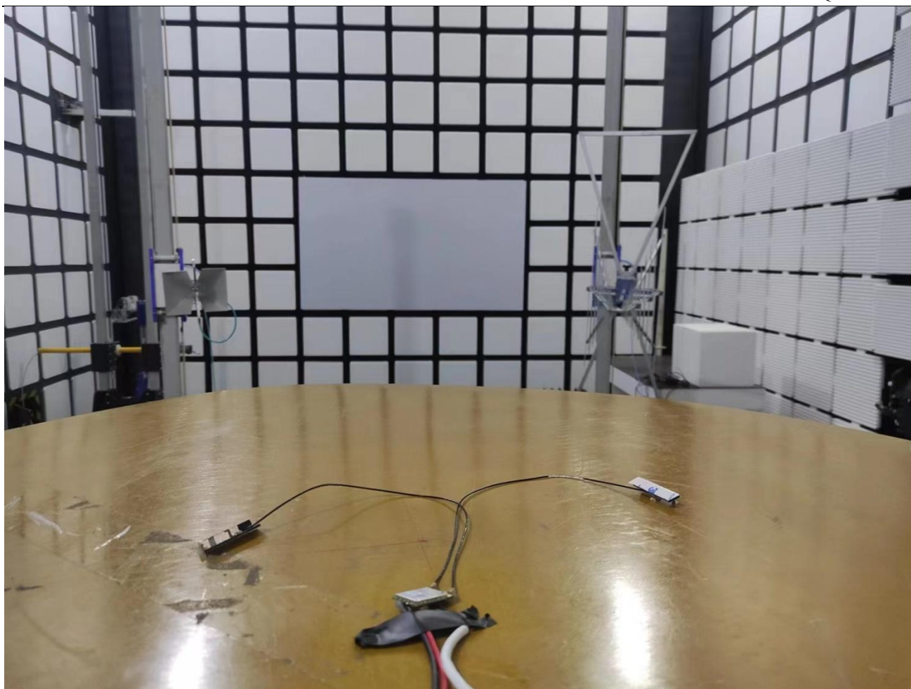
RSE
