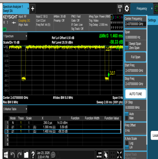
NTNV-11G-Ant1-2437
