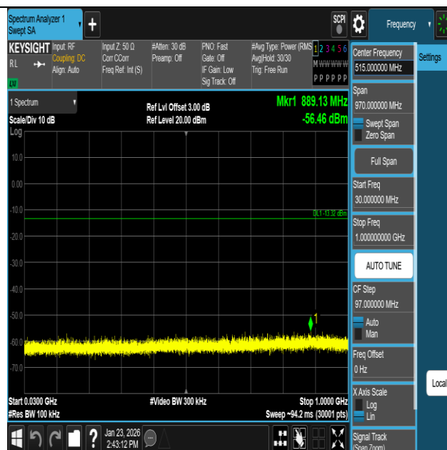
11G-Ant1-2412-30~1000-PASS
