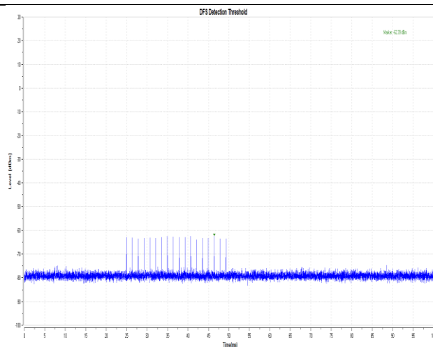
11AC80SISO-5290-Type0-PASS
