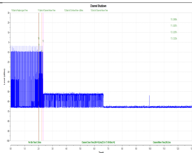
11AC80SISO-5290-Type0-PASS
