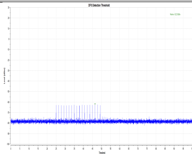
11AC80SISO-5530-Type0-PASS
