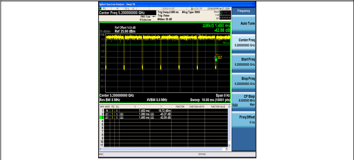
NTNV-11A-Ant1-5200
