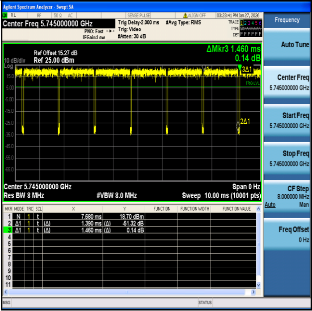
NTNV-11A-Ant1-5745
