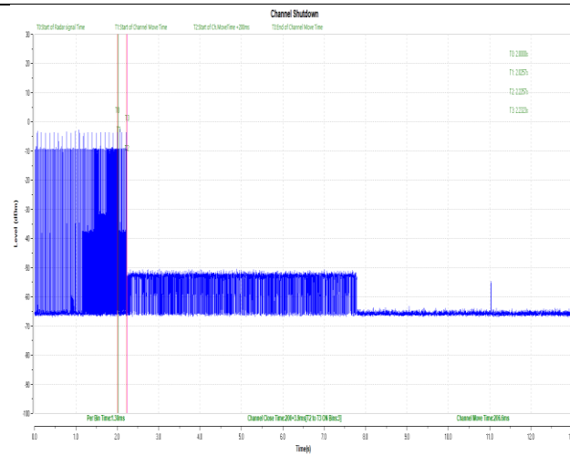
11AC80SISO-5290-Type0-PASS
