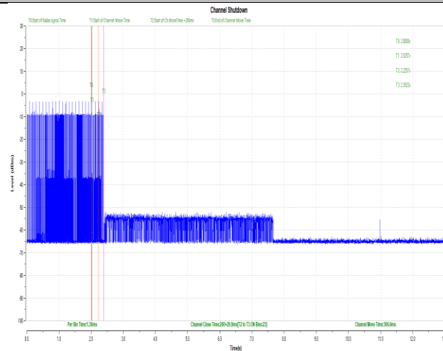
11AC80SISO-5530-Type0-PASS
