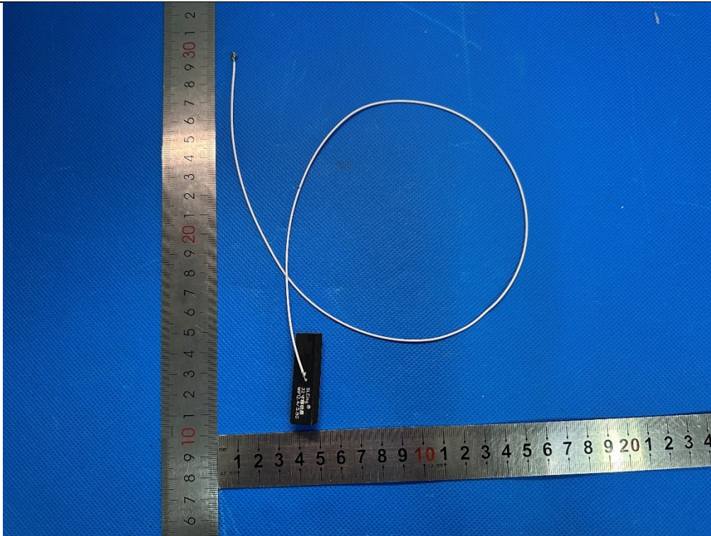
EUT Photo(10) Wi-Fi ANT2
