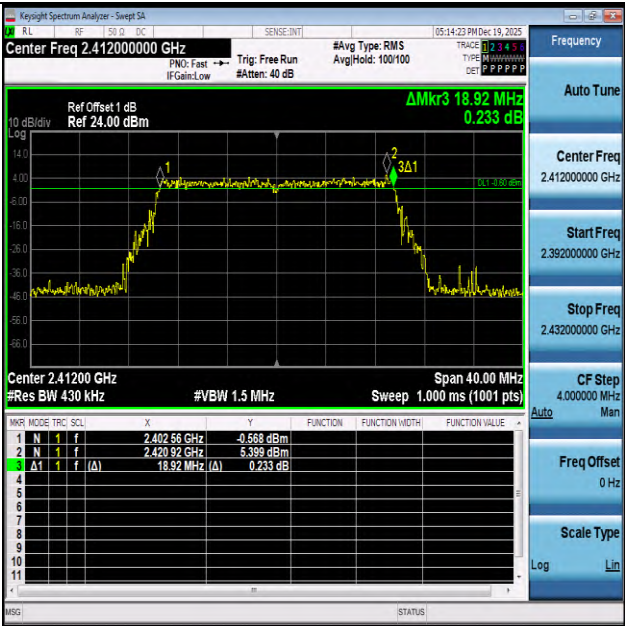
11AX20-2412-PASS
