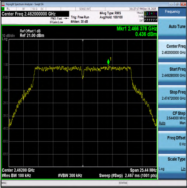
11G-2462-PASS
