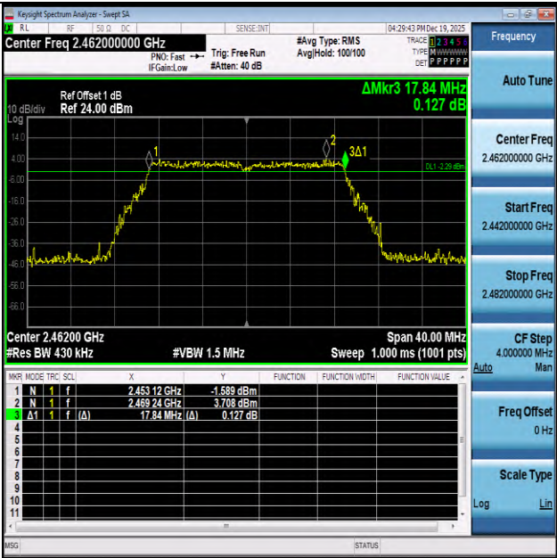
11N20-2462-PASS
