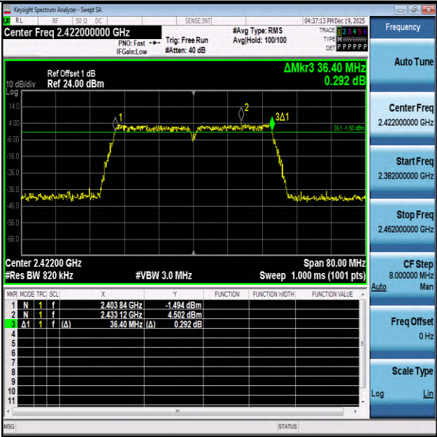
11N40-2422-PASS
