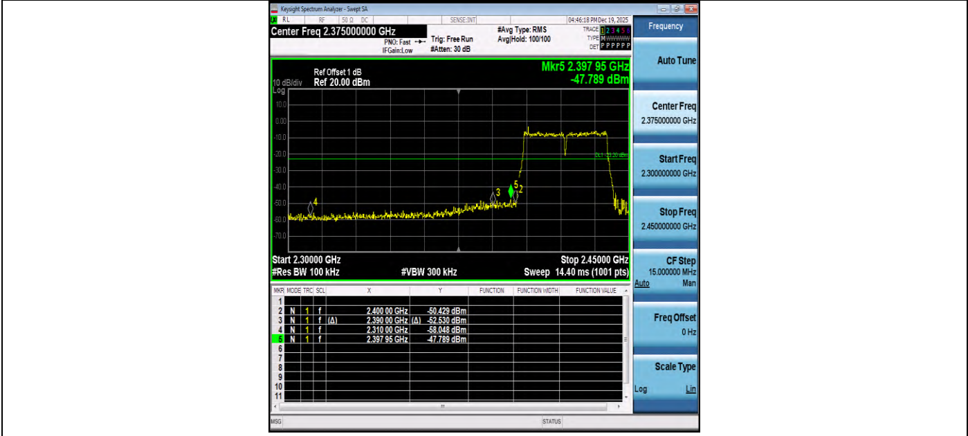
11N40-2422-PASS
