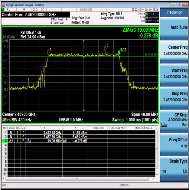
11AX20-2462-PASS
