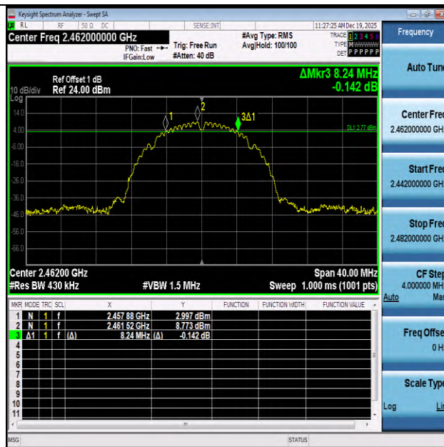
11B-2462-PASS
