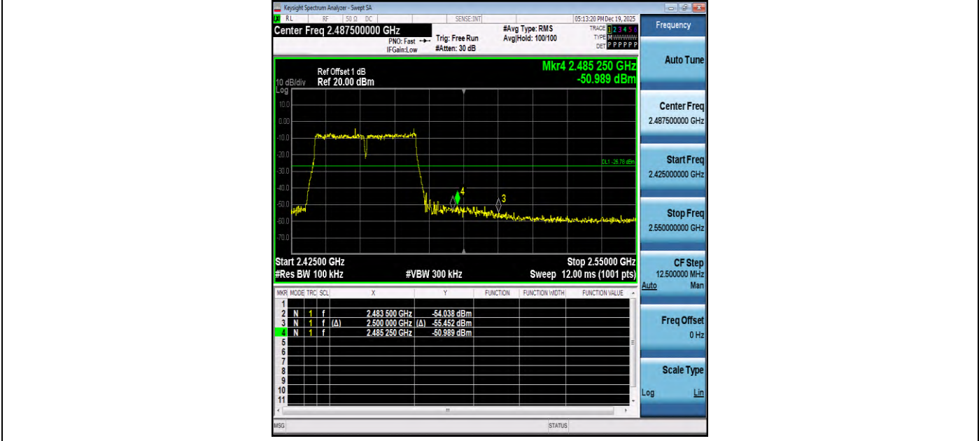
11N40-2452-PASS
