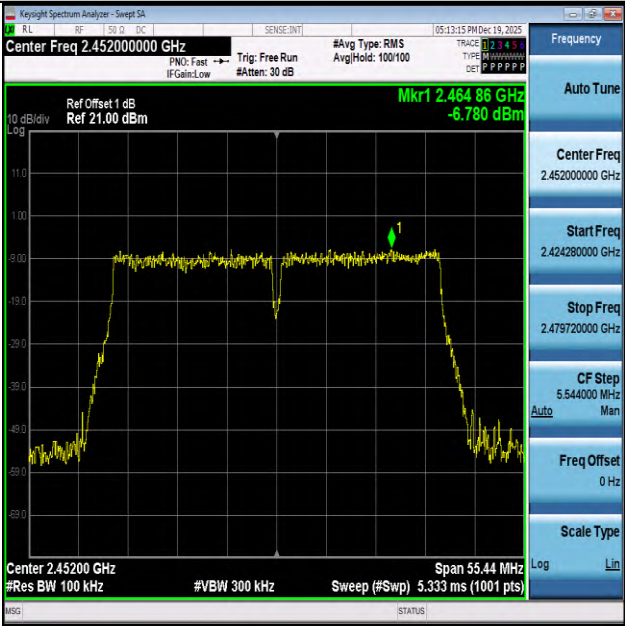
11N40-2452-PASS
