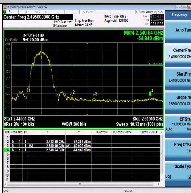
11B-2462-PASS
