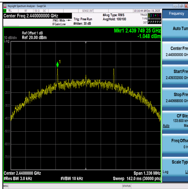
BLE_500K-2440-PASS
