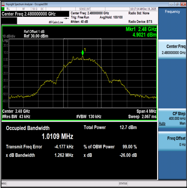
BLE_500K-2480
