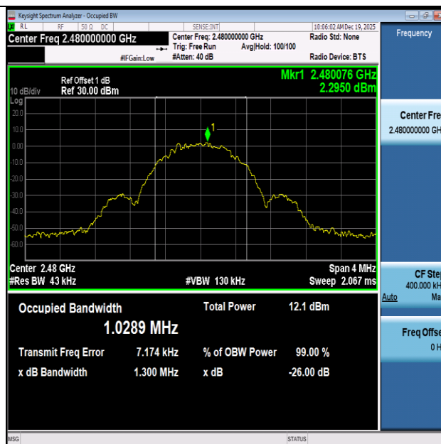
BLE 1M-2480
