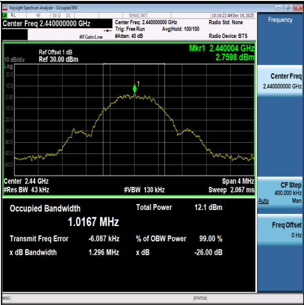
BLE_500K-2440
