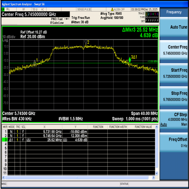
11A-Ant1-5745
