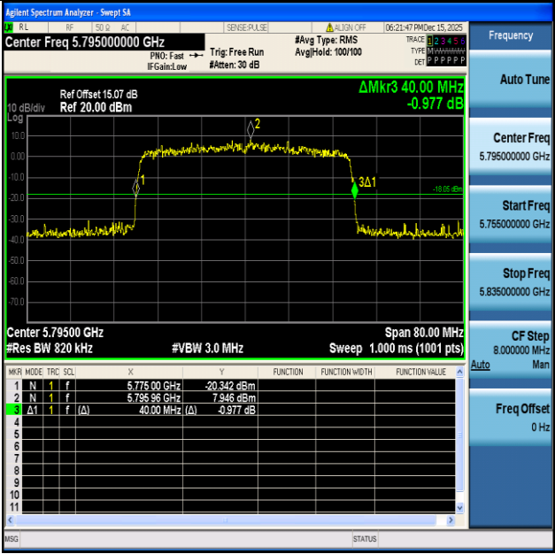
11AX40ISO-Ant1-5795
