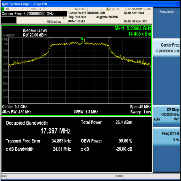
11A-Ant1-5200
