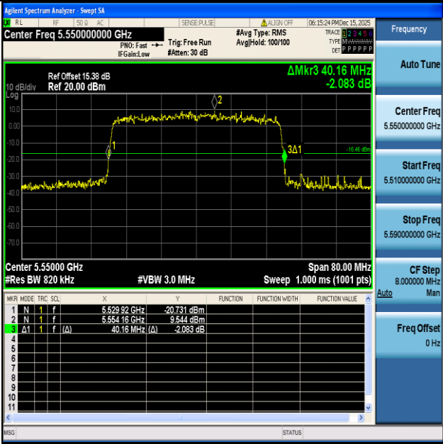
11AX40ISO-Ant1-5550
