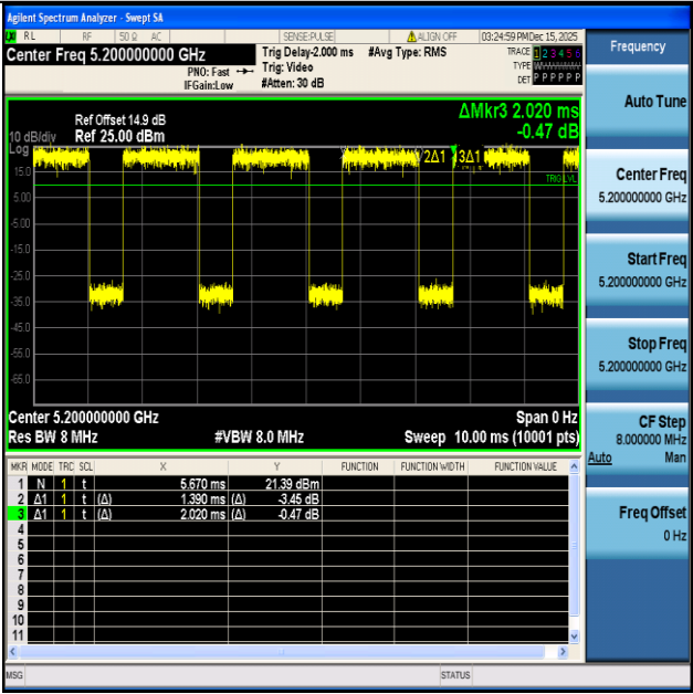
NTVN-11A-Ant1-5200
