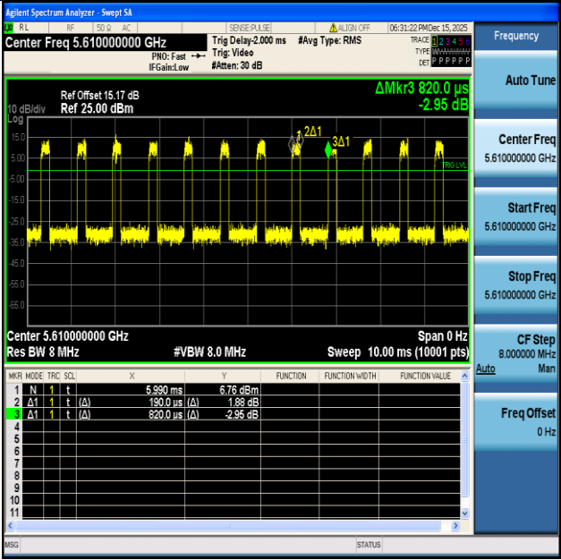
NTNV-11AX80SISO-Ant1-5610
