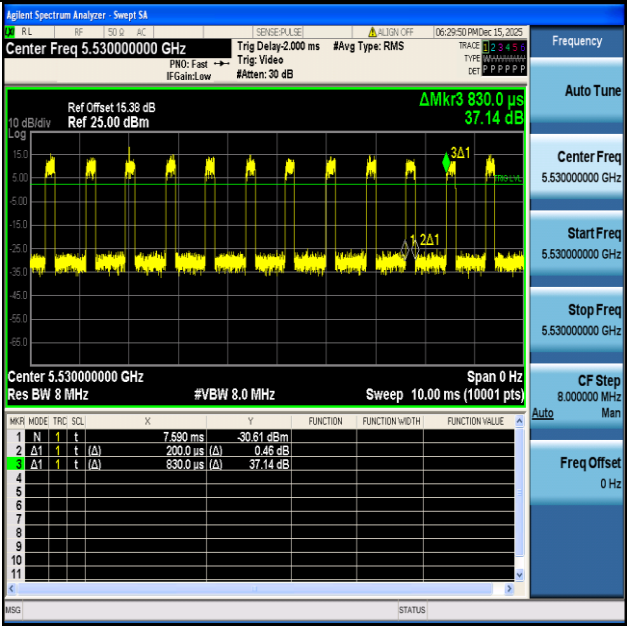
NTNV-11AX80SISO-Ant1-5530
