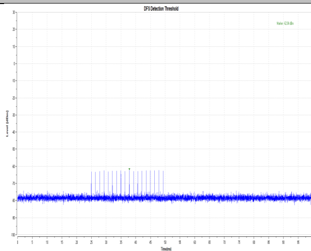
11AC80SISO-5530-Type0-PASS
