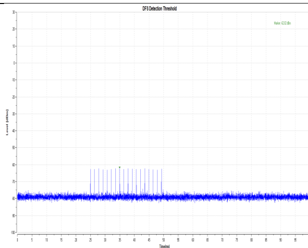
11AC80SISO-5290-Type0-PASS
