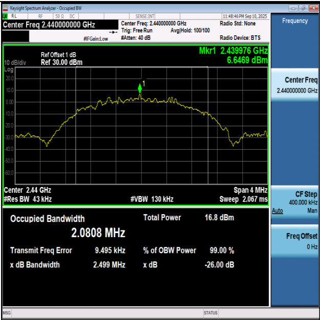
BLE_2M-Ant1-2440
