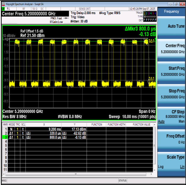
NTNV-11BE20SISO-Ant1-5200
