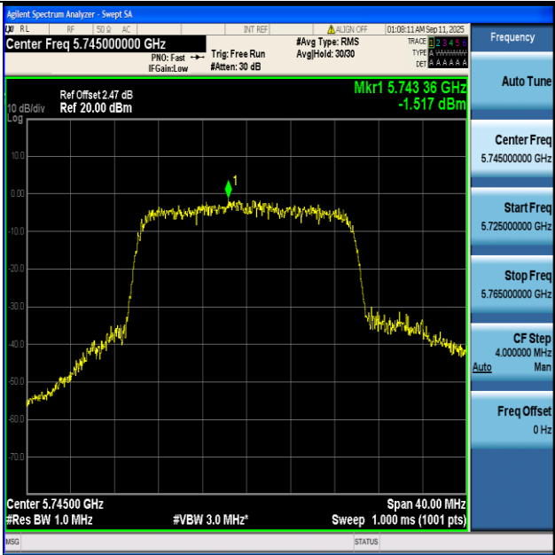
11BE20-Ant1+2-5745-PASS
