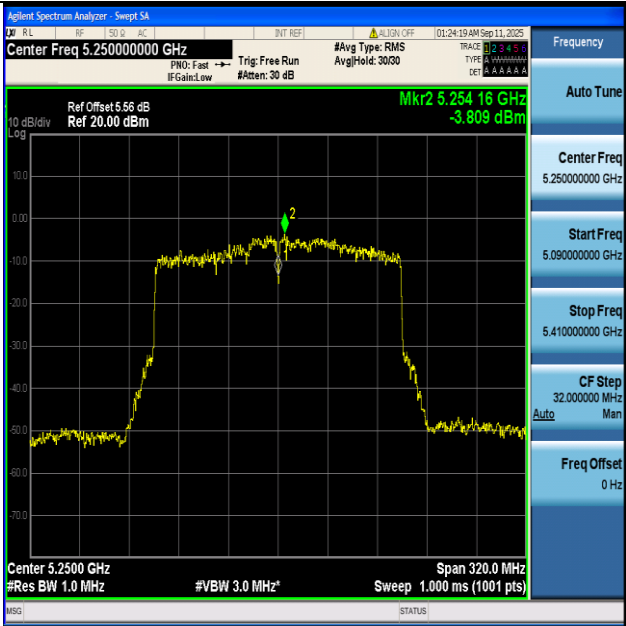
11BE160-Ant1+2-5250_UNII-2A-PASS
