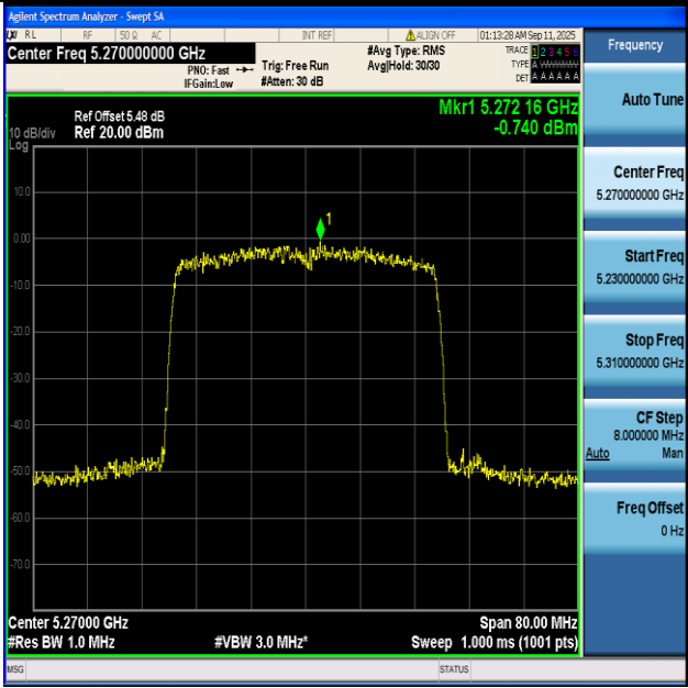
11BE40-Ant1+2-5270-PASS
