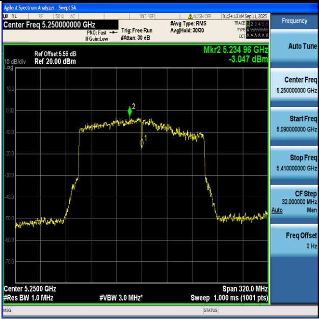
11BE160-Ant1+2-5250_UNII-1-PASS
