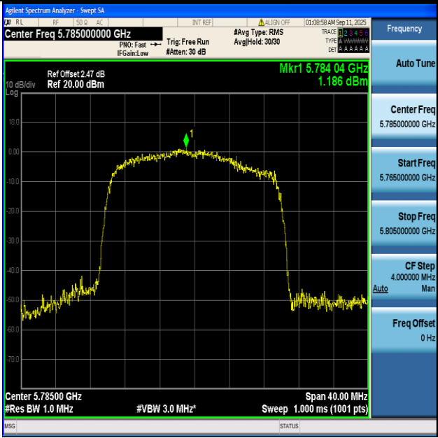
11BE20-Ant1+2-5785-PASS
