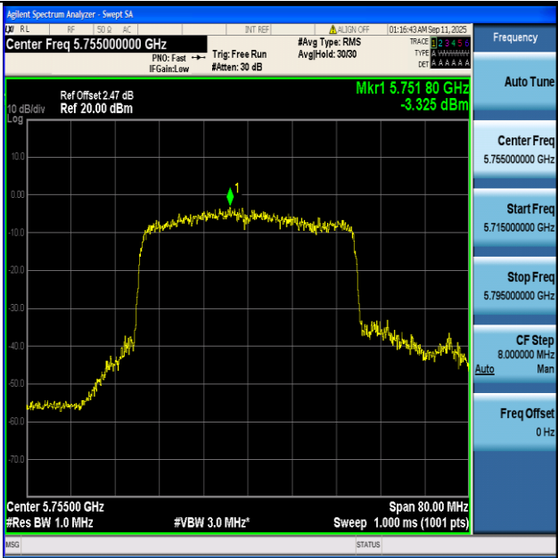
11BE40-Ant1+2-5755-PASS
