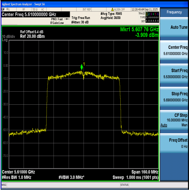
11AC80-Ant1+2-5610-PASS
