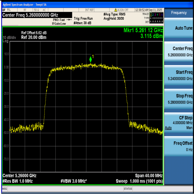
11AX20-Ant1+2-5260-PASS
