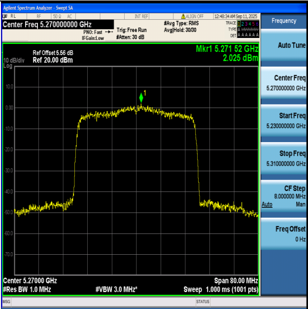
11AX40-Ant1+2-5270-PASS
