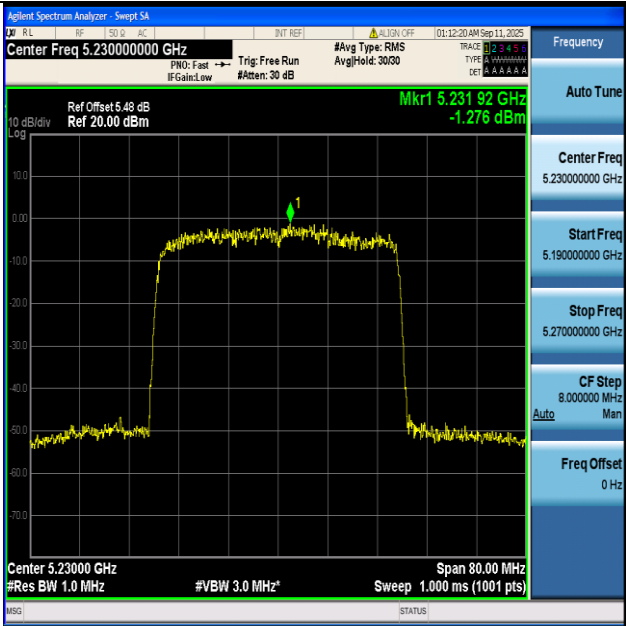
11BE40-Ant1+2-5230-PASS
