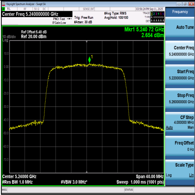
11BE20-Ant1+2-5240-PASS
