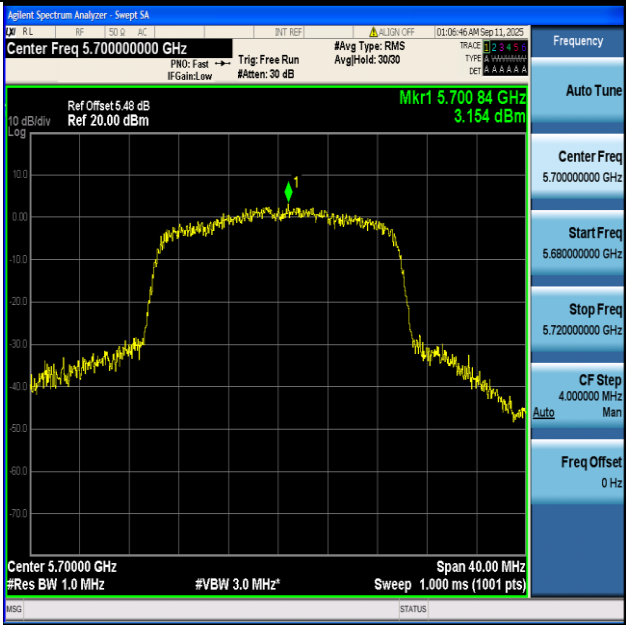
11BE20-Ant1+2-5700-PASS
