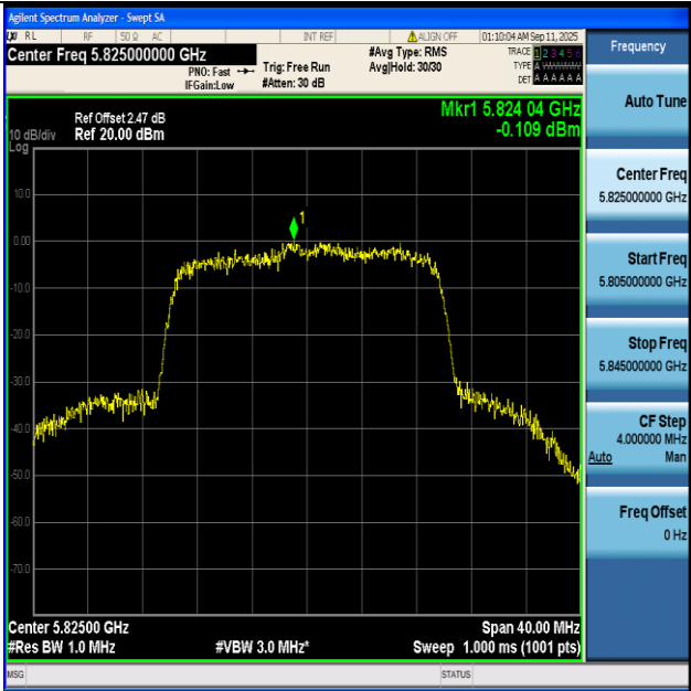
11BE20-Ant1+2-5825-PASS
