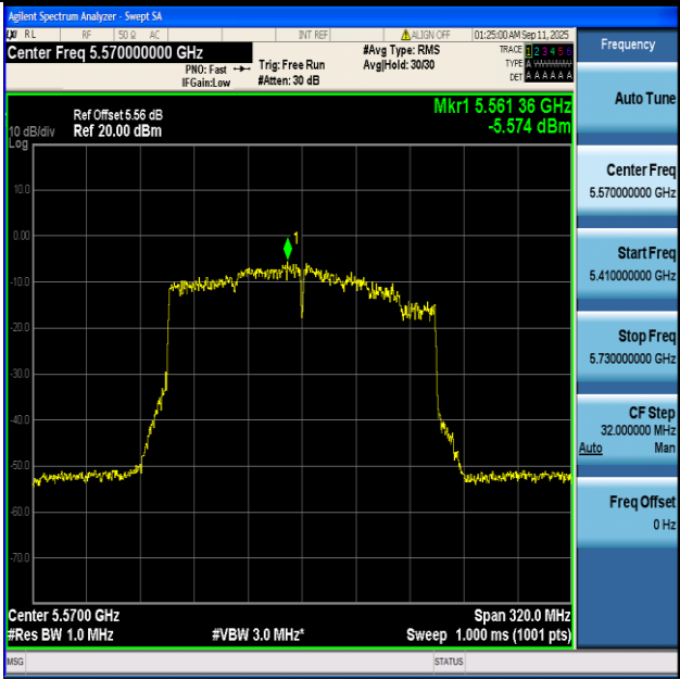
11BE160-Ant1+2-5570-PASS
