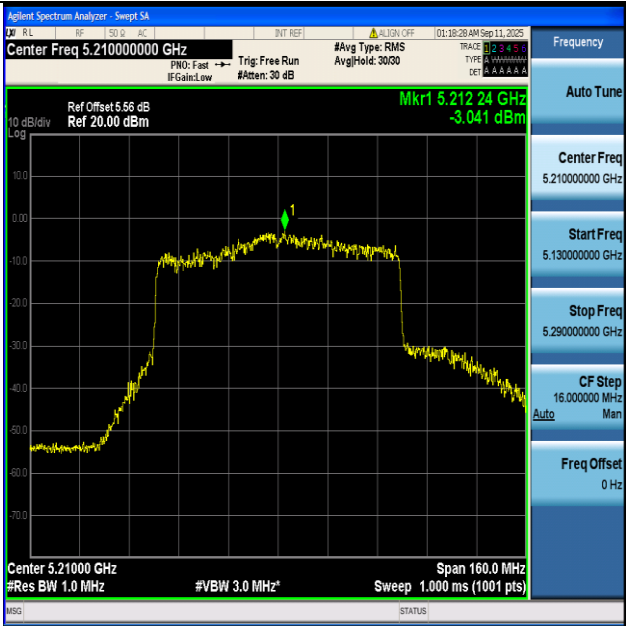
11BE80-Ant1+2-5210-PASS
