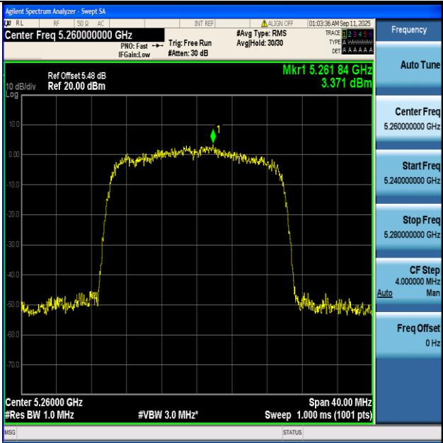
11BE20-Ant1+2-5260-PASS
