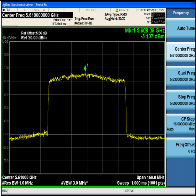
11BE80-Ant1+2-5610-PASS
