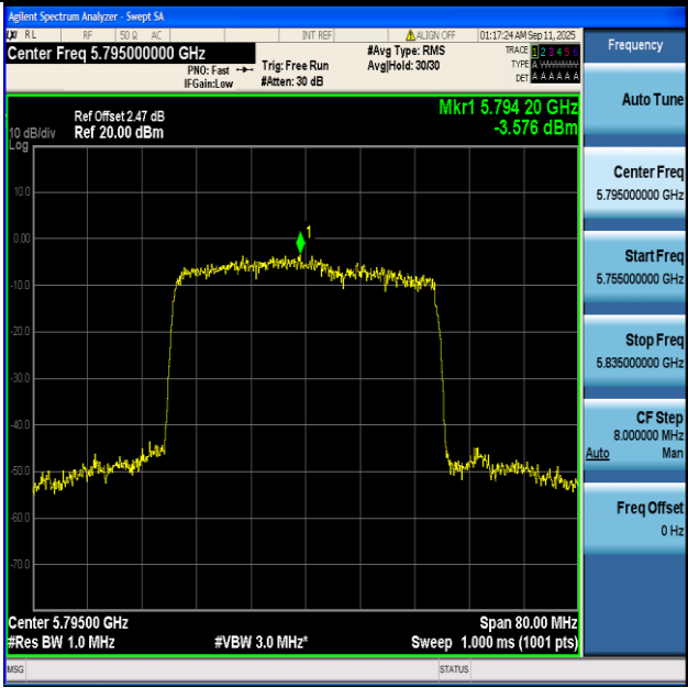
11BE40-Ant1+2-5795-PASS
