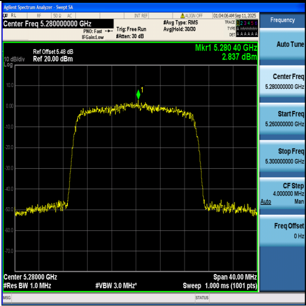
11BE20-Ant1+2-5280-PASS
