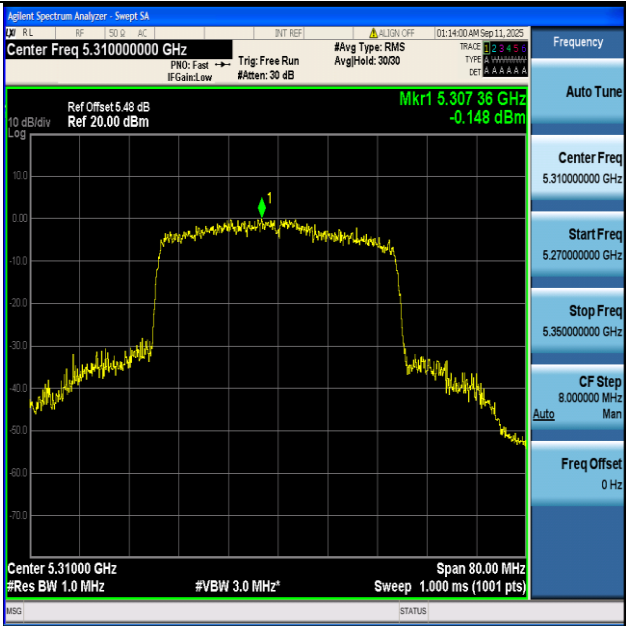
11BE40-Ant1+2-5310-PASS
