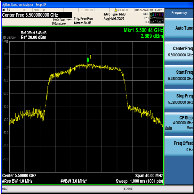
11BE20-Ant1+2-5500-PASS
