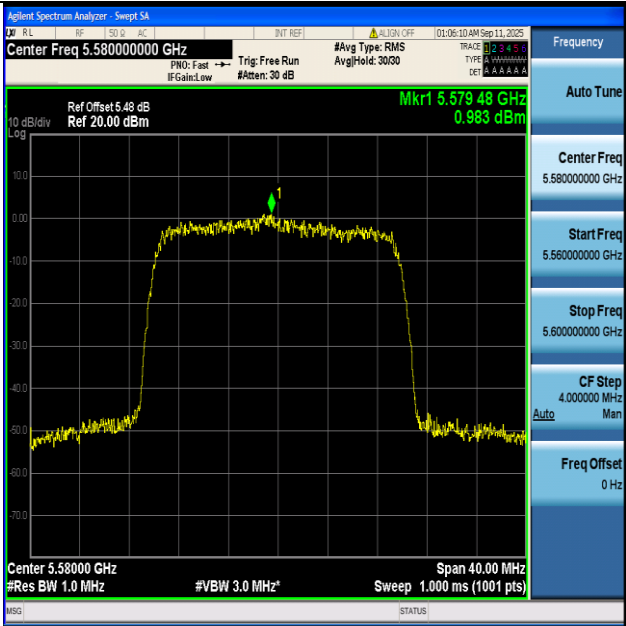
11BE20-Ant1+2-5580-PASS
