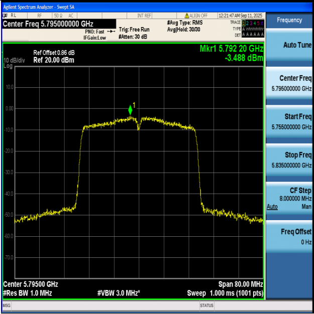
11AC40-Ant1+2-5795-PASS
