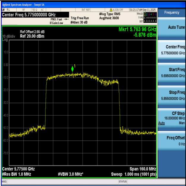
11BE80-Ant1+2-5775-PASS
