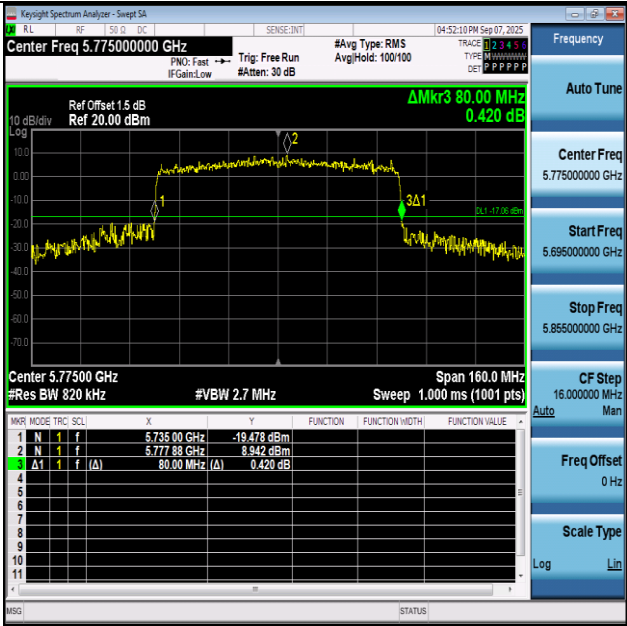
11BE80SISO-Ant1-5775
