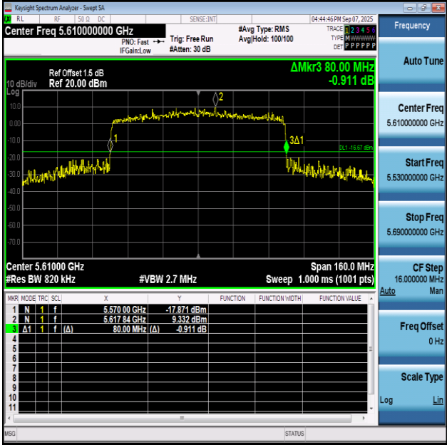
11BE80SISO-Ant1-5610
