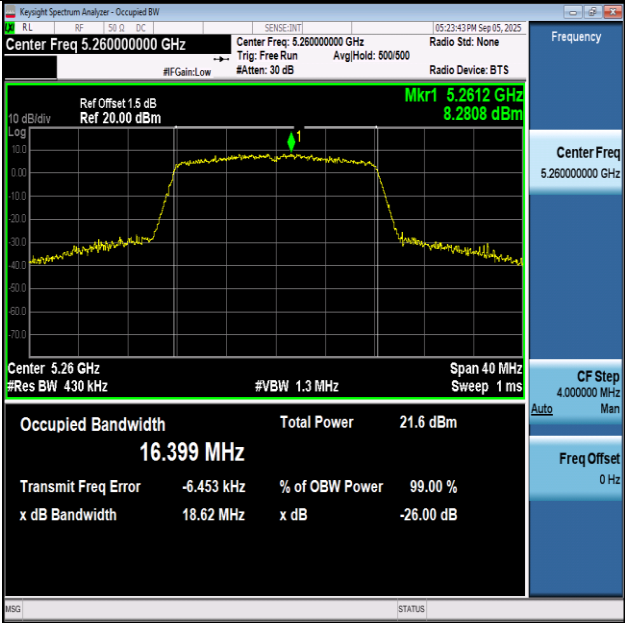
11A-Ant1-5260
