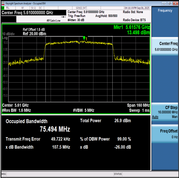
11AC80SISO-Ant1-5610
