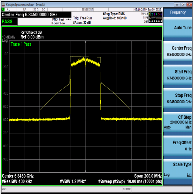
NTVN-11AX40-Ant1+2-6845-PASS
