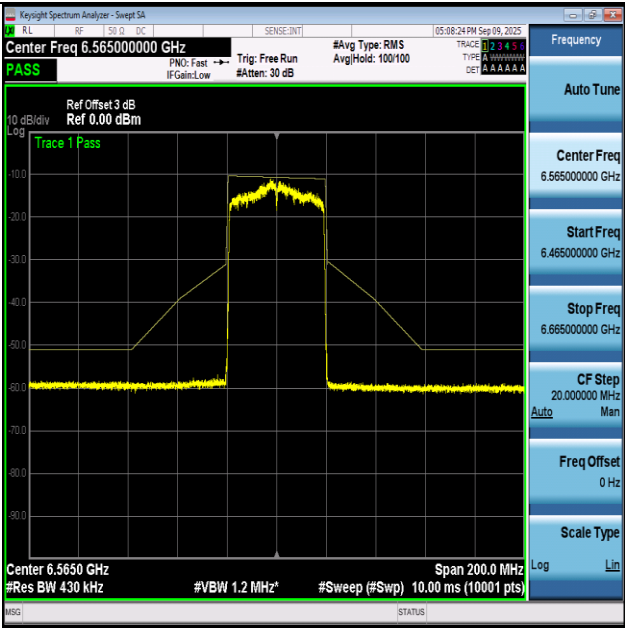
NTVN-11AX40-Ant1+2-6565-PASS
