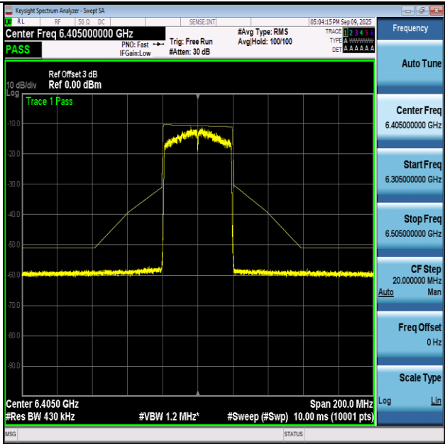
NTVN-11AX40-Ant1+2-6405-PASS
