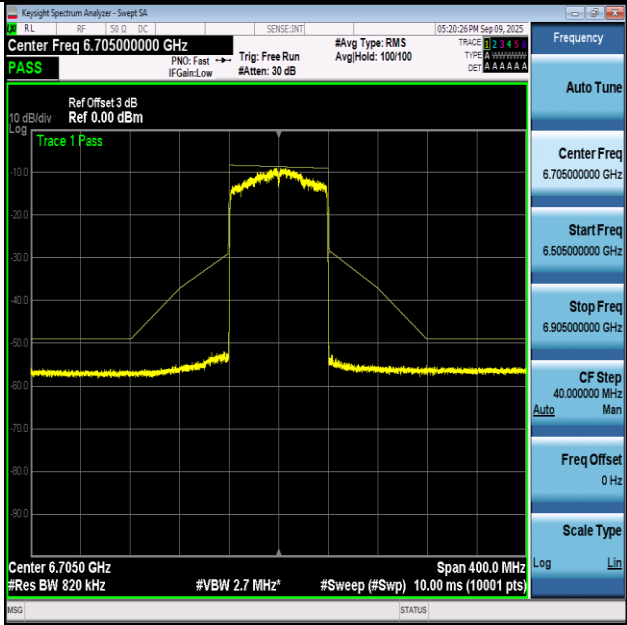
NTVN-11AX80-Ant1+2-6705-PASS
