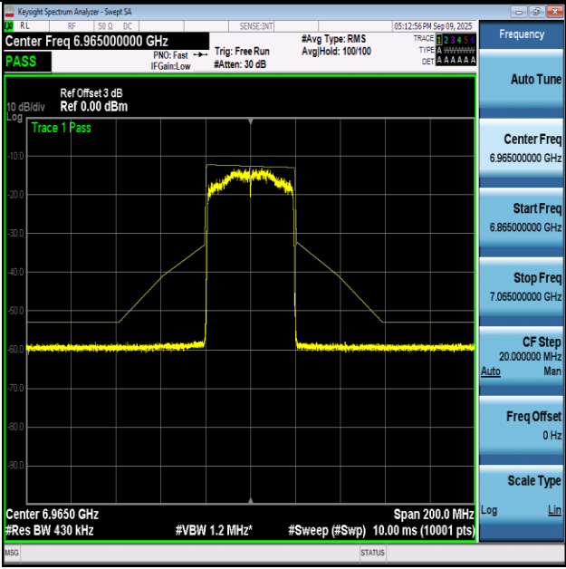
NTVN-11AX40-Ant1+2-6965-PASS
