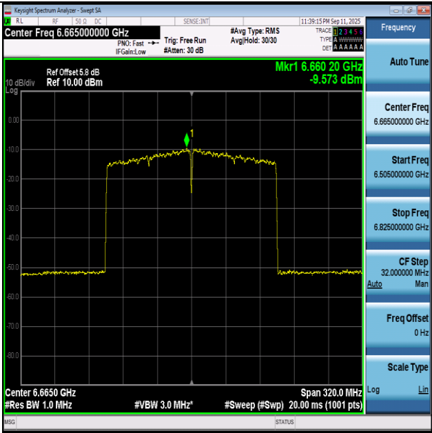
11BE160-Ant1+2-6665-PASS
