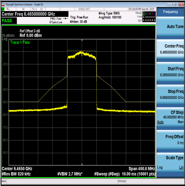
NTVN-11AX80-Ant1+2-6465-PASS
