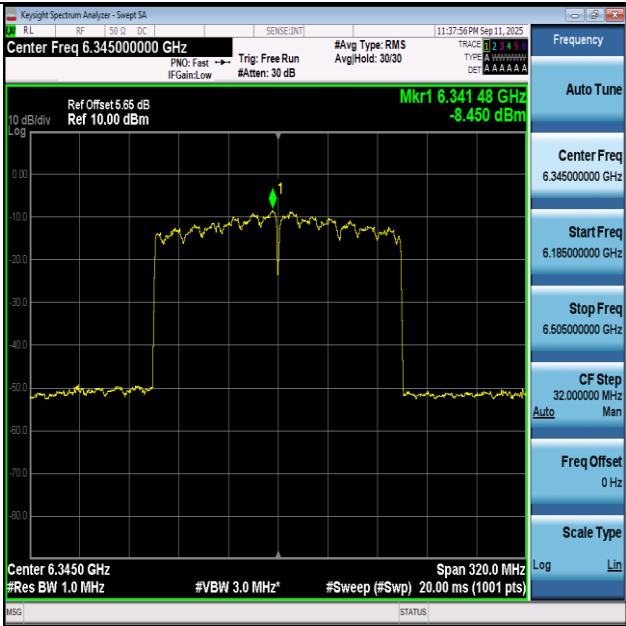
11BE160-Ant1+2-6345-PASS
