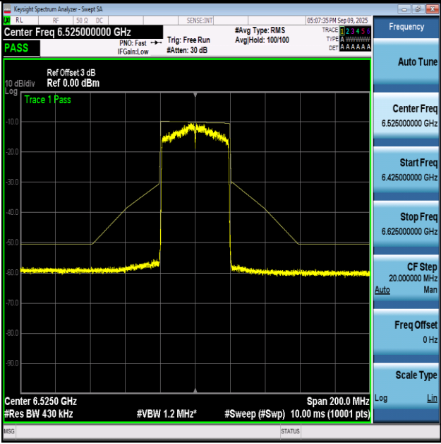
NTVN-11AX40-Ant1+2-6525-PASS
