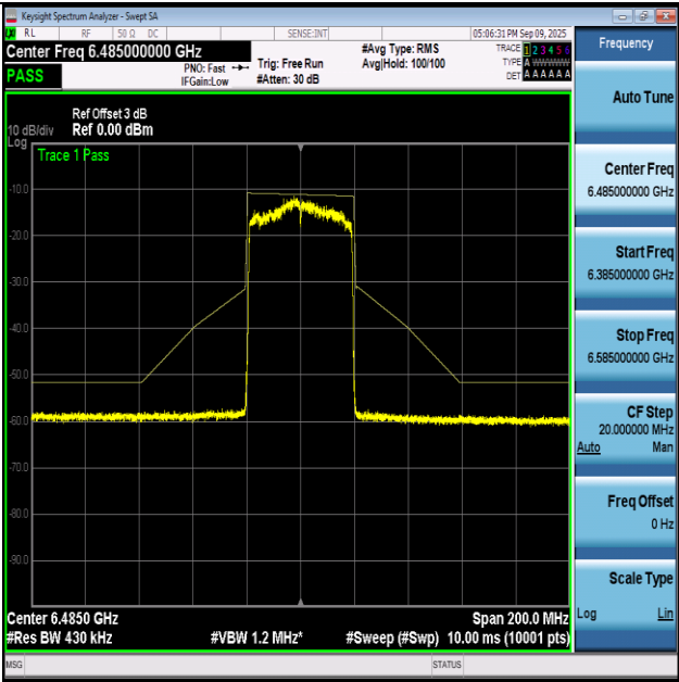
NTVN-11AX40-Ant1+2-6485-PASS
