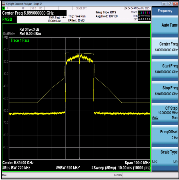
NTVN-11AX20-Ant1+2-6895-PASS
