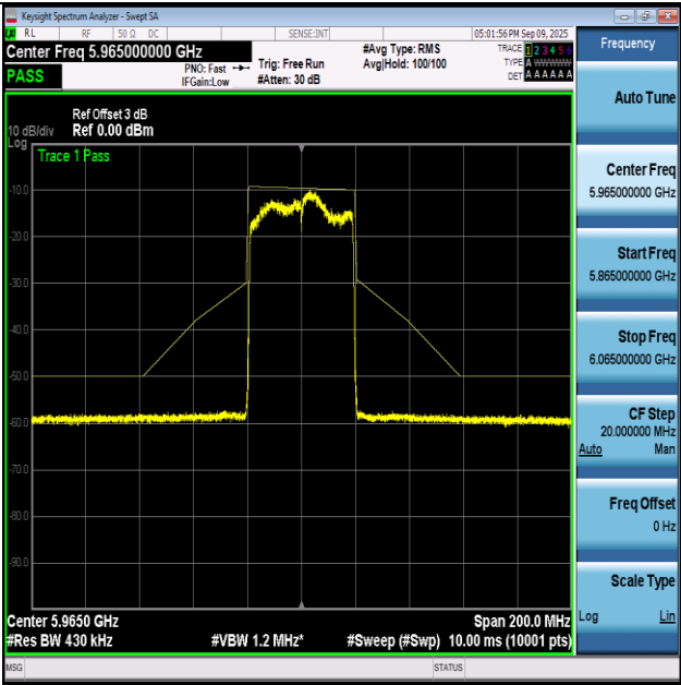
NTVN-11AX40-Ant1+2-5965-PASS
