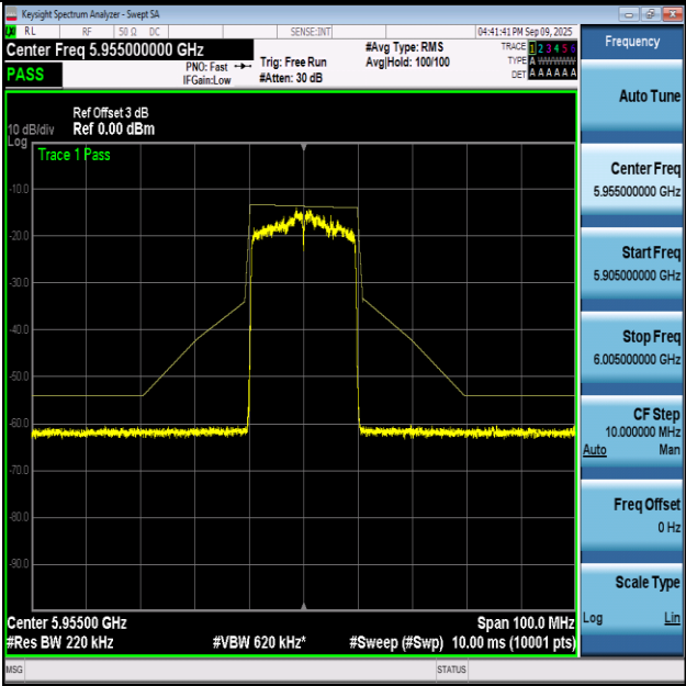
NTVN-11AX20-Ant1+2-5955-PASS
