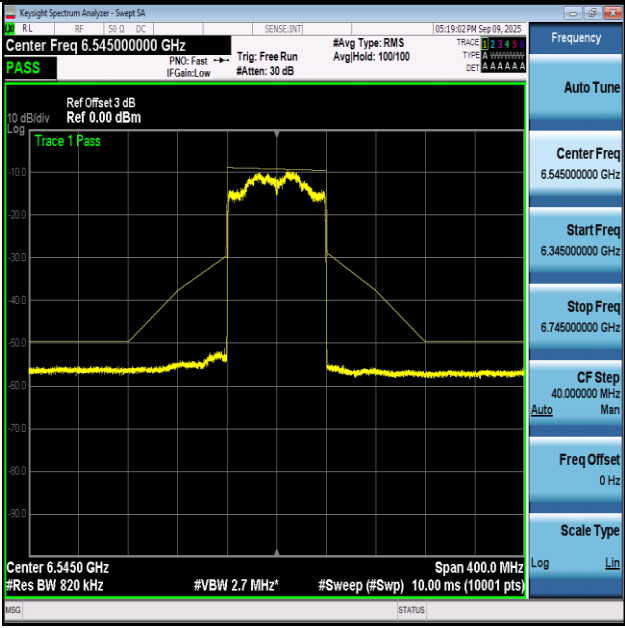
NTVN-11AX80-Ant1+2-6545-PASS
