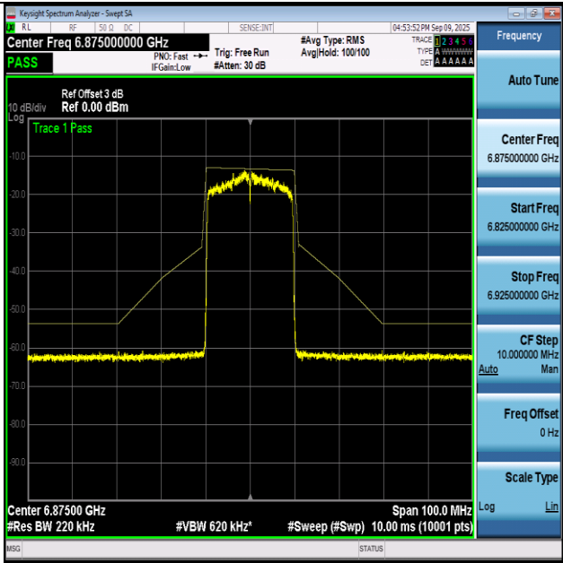
NTVN-11AX20-Ant1+2-6875-PASS
