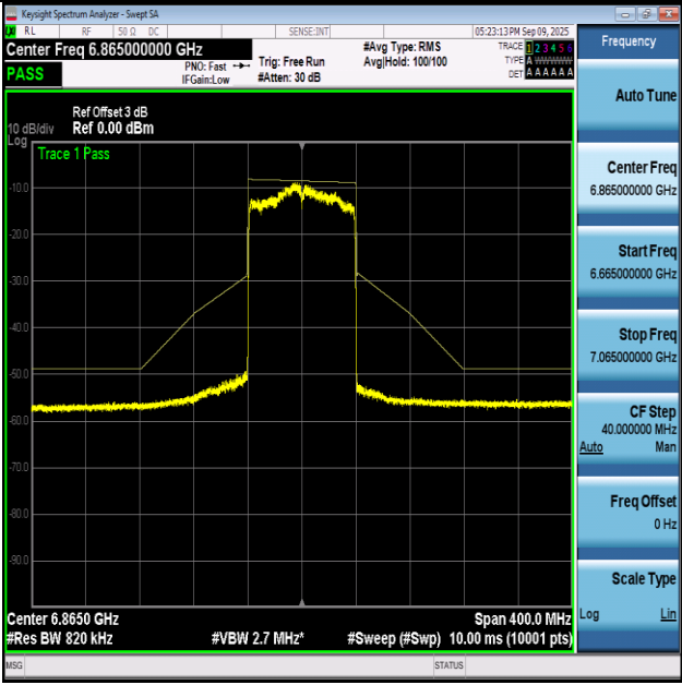
NTVN-11AX80-Ant1+2-6865-PASS
