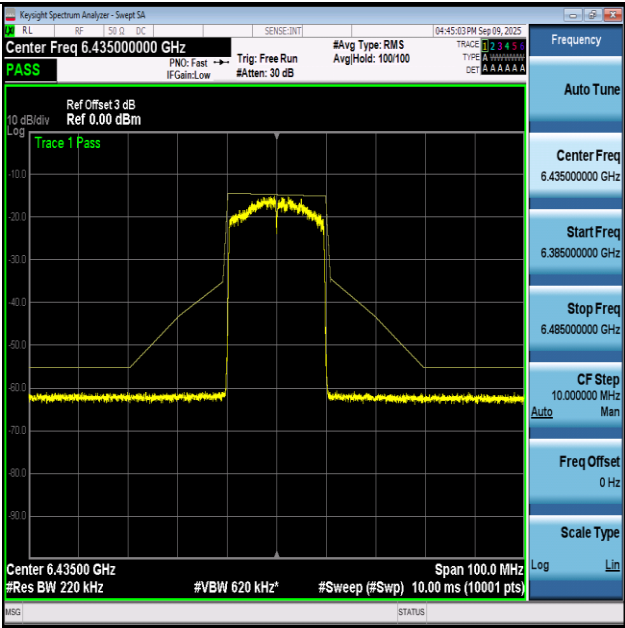
NTVN-11AX20-Ant1+2-6435-PASS
