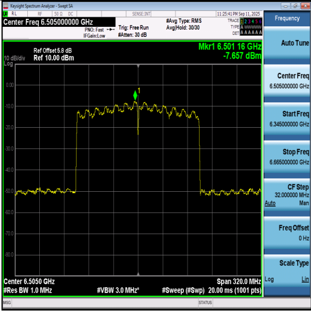
11BE160-Ant1+2-6505-PASS
