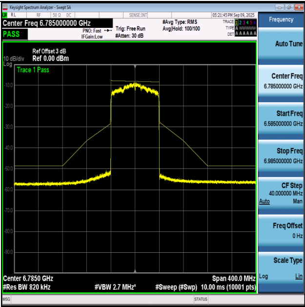
NTVN-11AX80-Ant1+2-6785-PASS
