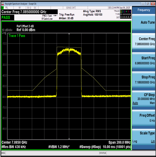
NTVN-11AX40-Ant1+2-7085-PASS
