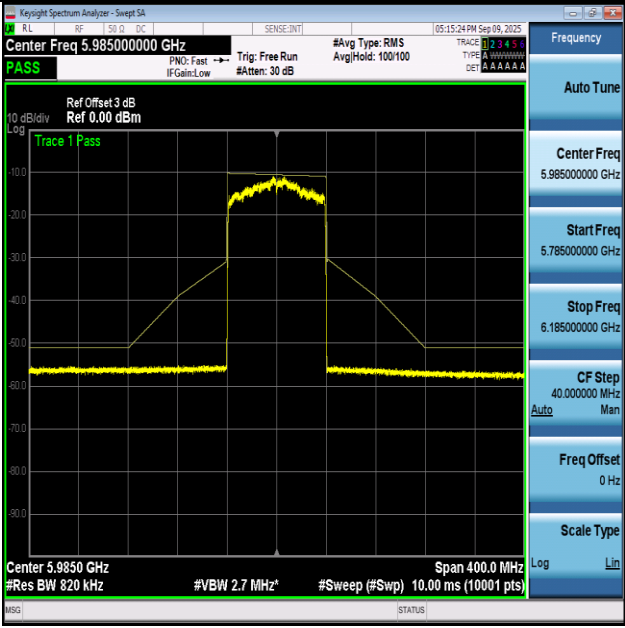
NTVN-11AX80-Ant1+2-5985-PASS
