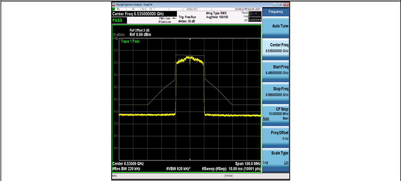
NTVN-11AX20-Ant1+2-6535-PASS
