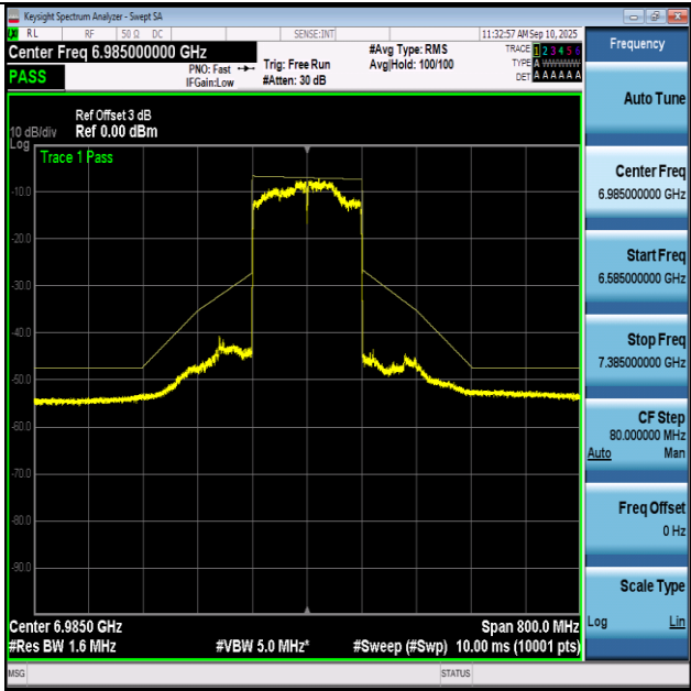
NTNV-11BE160-Ant1+2-6985-PASS
