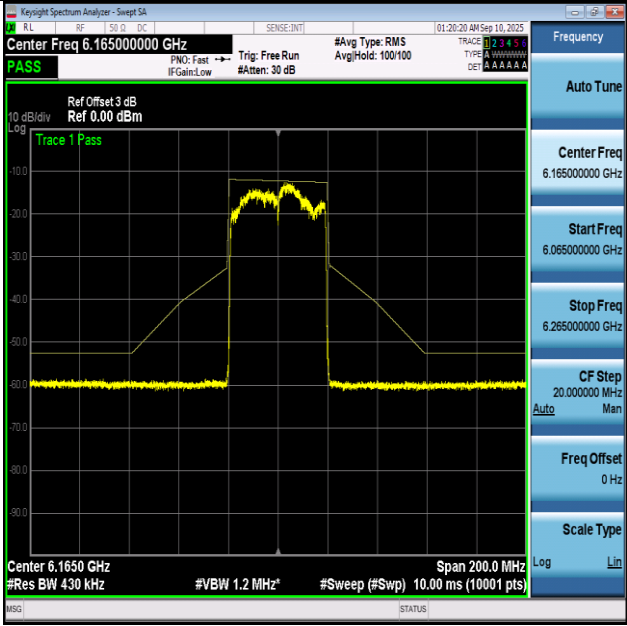
NTNV-11BE40-Ant1+2-6165-PASS
