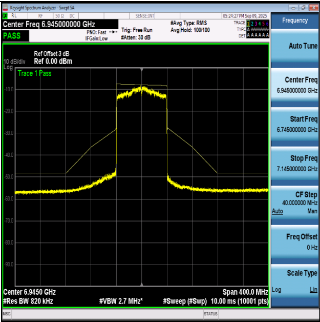
NTVN-11AX80-Ant1+2-6945-PASS
