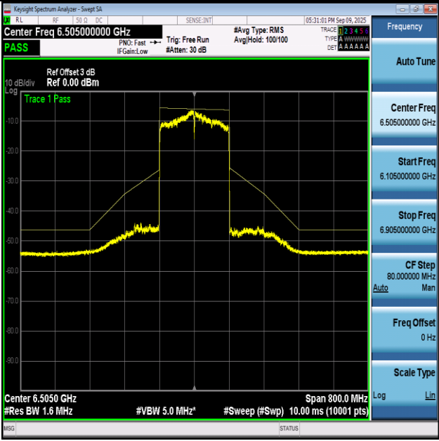
NTVN-11AX160-Ant1+2-6505-PASS
