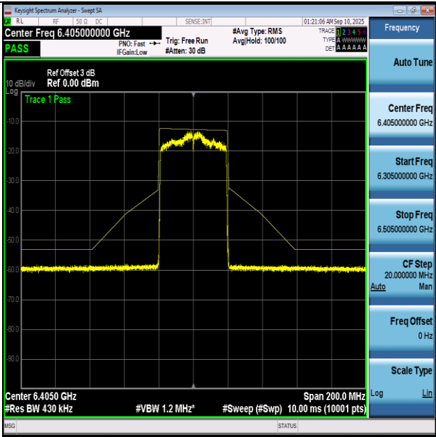
NTNV-11BE40-Ant1+2-6405-PASS
