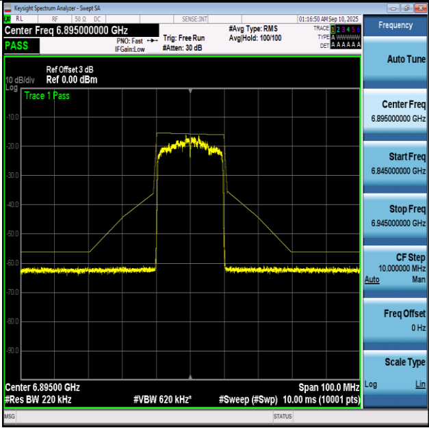
NTNV-11BE20-Ant1+2-6895-PASS
