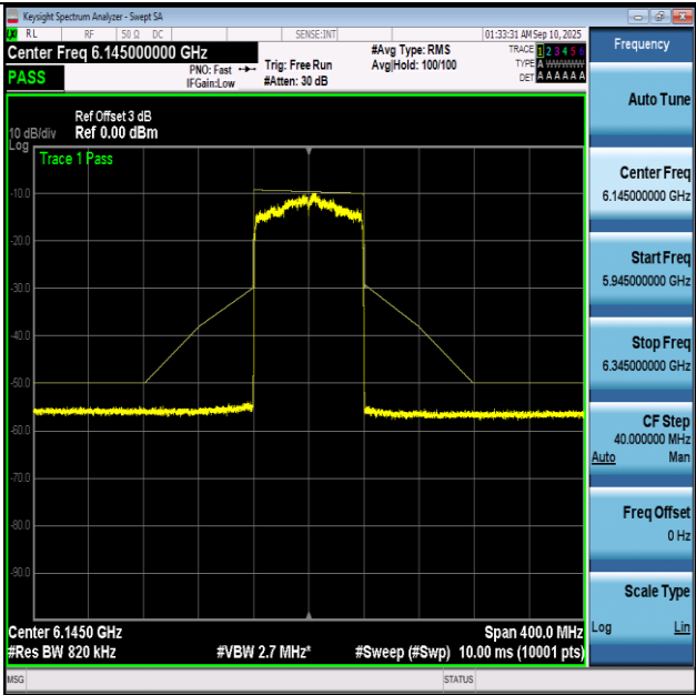
NTNV-11BE80-Ant1+2-6145-PASS
