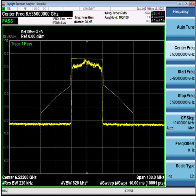
NTNV-11BE20-Ant1+2-6535-PASS
