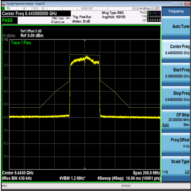
NTNV-11BE40-Ant1+2-6445-PASS
