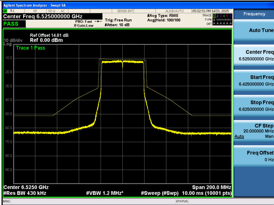
NTNV-11AX40-Ant1-6925-PASS
