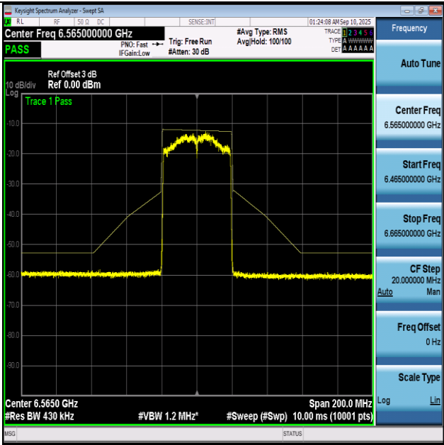
NTNV-11BE40-Ant1+2-6565-PASS
