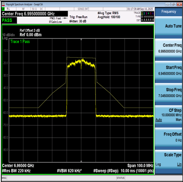
NTNV-11BE20-Ant1+2-6995-PASS
