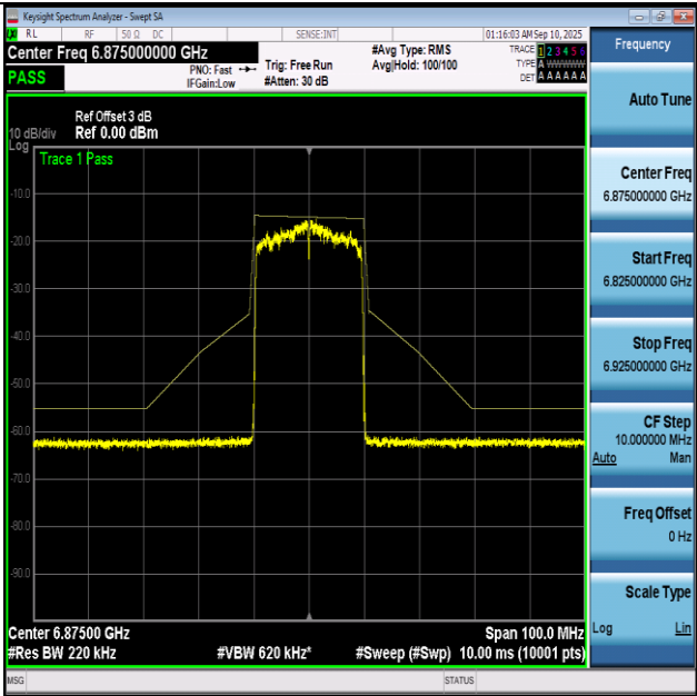
NTNV-11BE20-Ant1+2-6875-PASS
