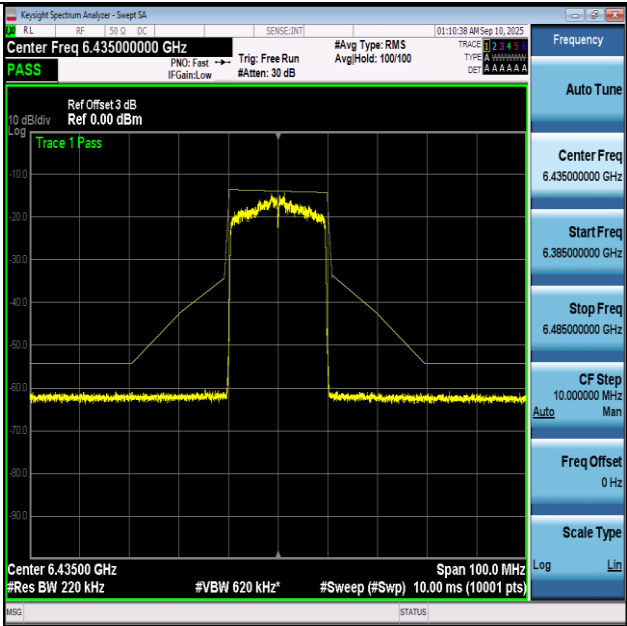
NTNV-11BE20-Ant1+2-6435-PASS
