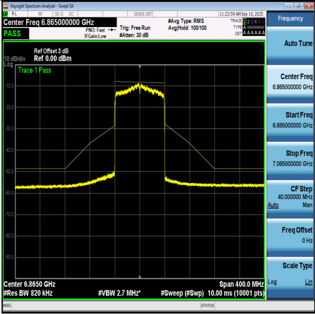
NTNV-11BE80-Ant1+2-6865-PASS
