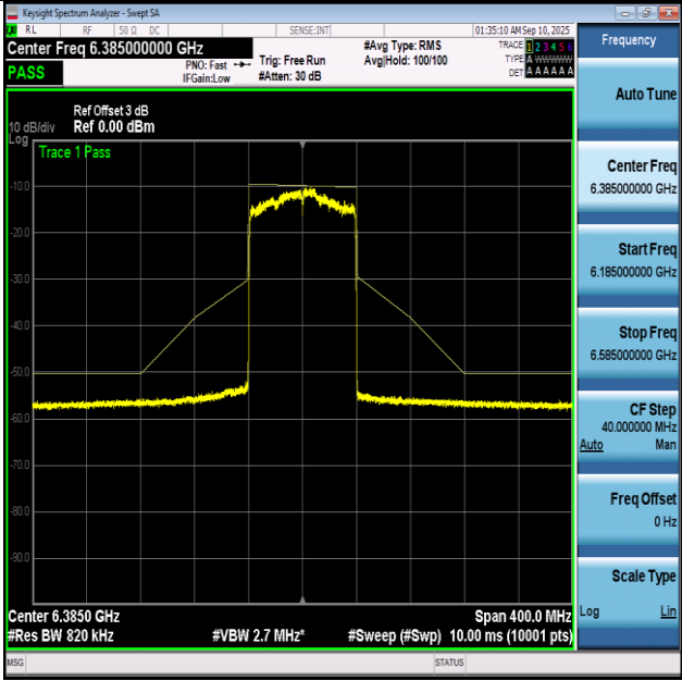
NTNV-11BE80-Ant1+2-6385-PASS
