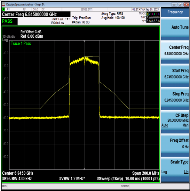
NTNV-11BE40-Ant1+2-6845-PASS
