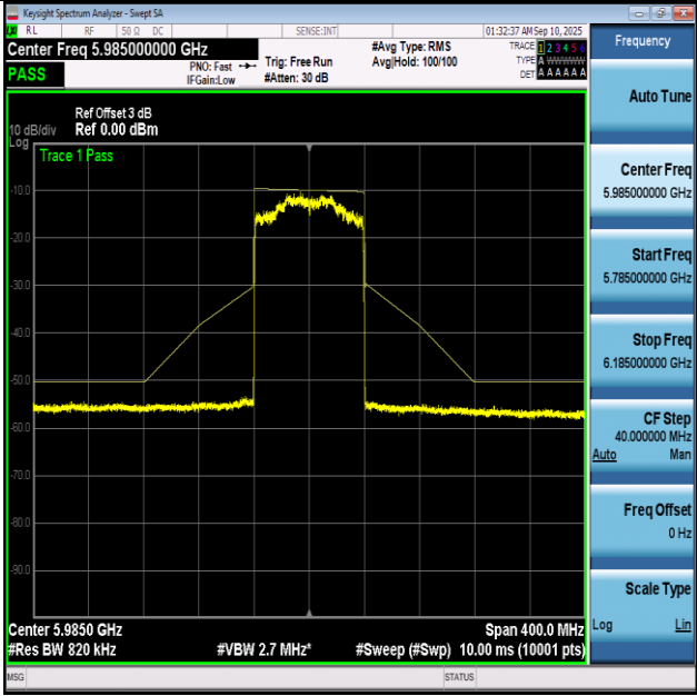
NTNV-11BE80-Ant1+2-5985-PASS
