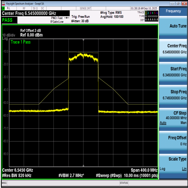
NTNV-11BE80-Ant1+2-6545-PASS
