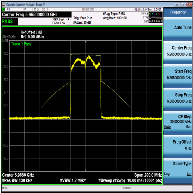
NTNV-11BE40-Ant1+2-5965-PASS
