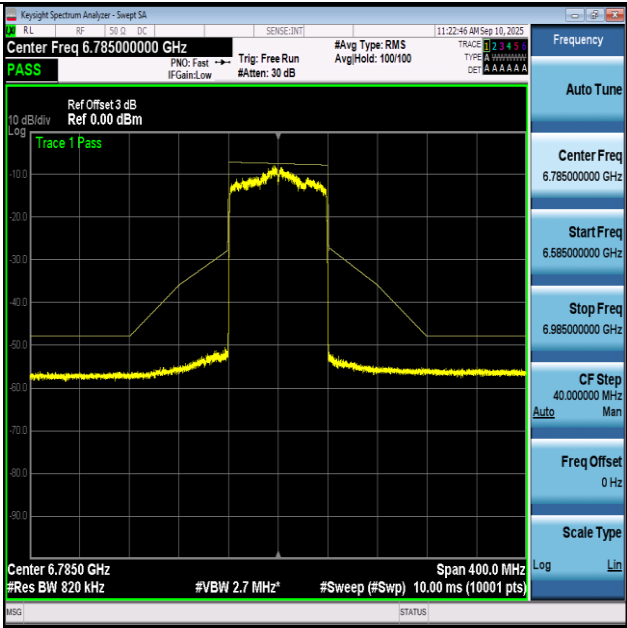
NTNV-11BE80-Ant1+2-6785-PASS
