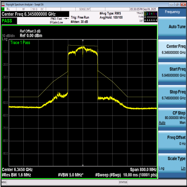
NTVN-11AX160-Ant1+2-6345-PASS
