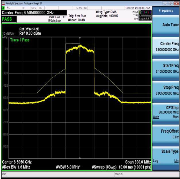
NTNV-11BE160-Ant1+2-6505-PASS
