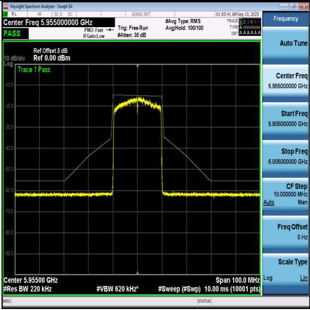
NTVN-11BE20-Ant1+2-5955-PASS
