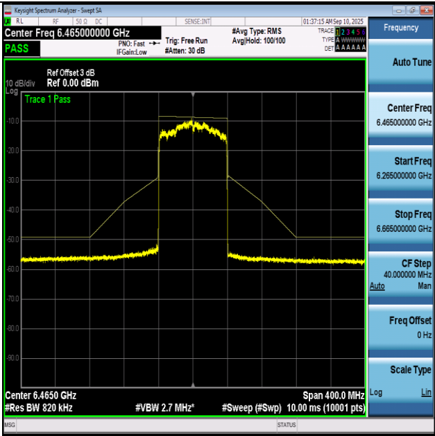
NTNV-11BE80-Ant1+2-6465-PASS
