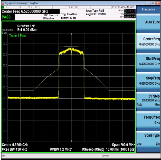
NTNV-11BE40-Ant1+2-6525-PASS
