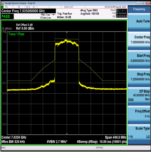
NTVN-11AX80-Ant1+2-7025-PASS
