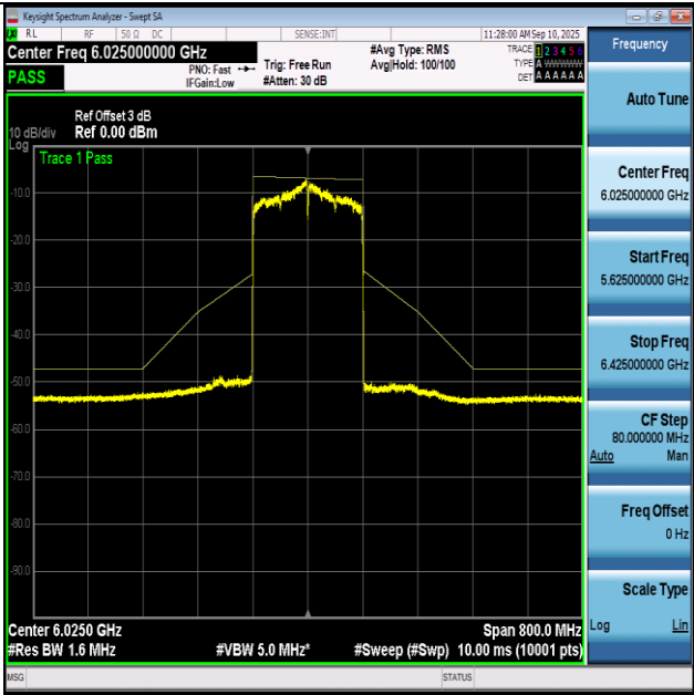
NTNV-11BE160-Ant1+2-6025-PASS
