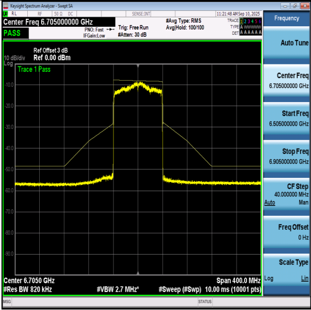
NTNV-11BE80-Ant1+2-6705-PASS
