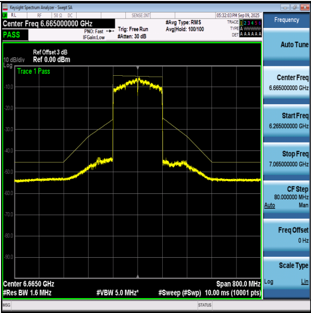
NTVN-11AX160-Ant1+2-6665-PASS
