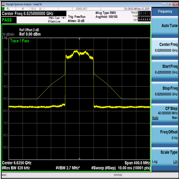
NTNV-11BE80-Ant1+2-6625-PASS
