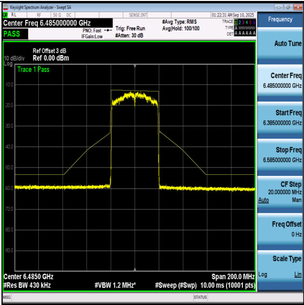
NTNV-11BE40-Ant1+2-6485-PASS
