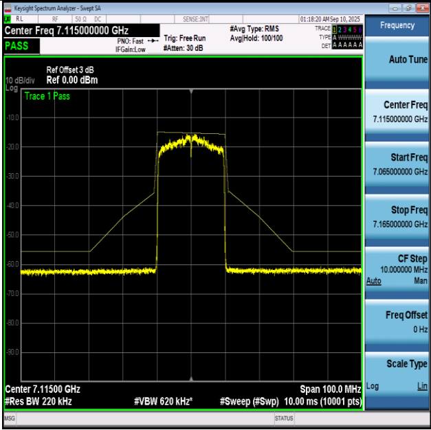
NTNV-11BE20-Ant1+2-7115-PASS
