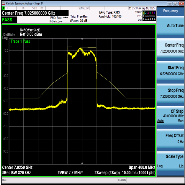
NTNV-11BE80-Ant1+2-7025-PASS
