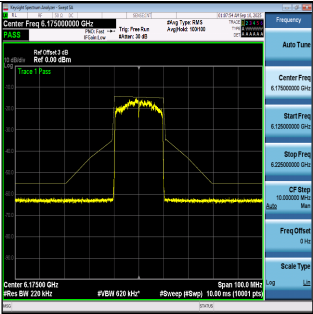
NTNV-11BE20-Ant1+2-6175-PASS
