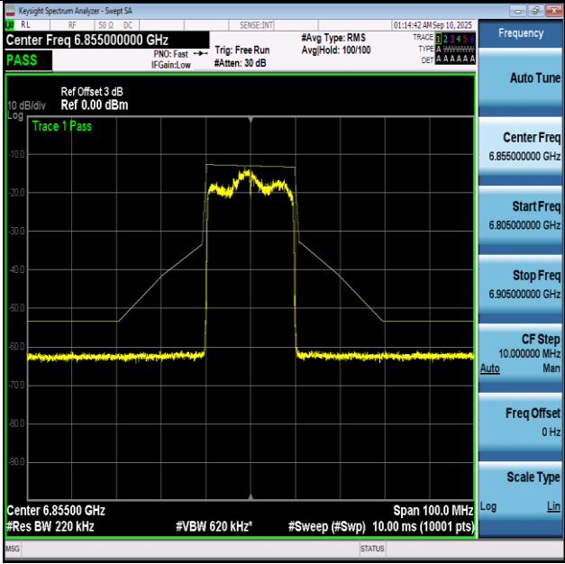
NTNV-11BE20-Ant1+2-6855-PASS
