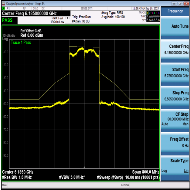
NTNV-11BE160-Ant1+2-6185-PASS
