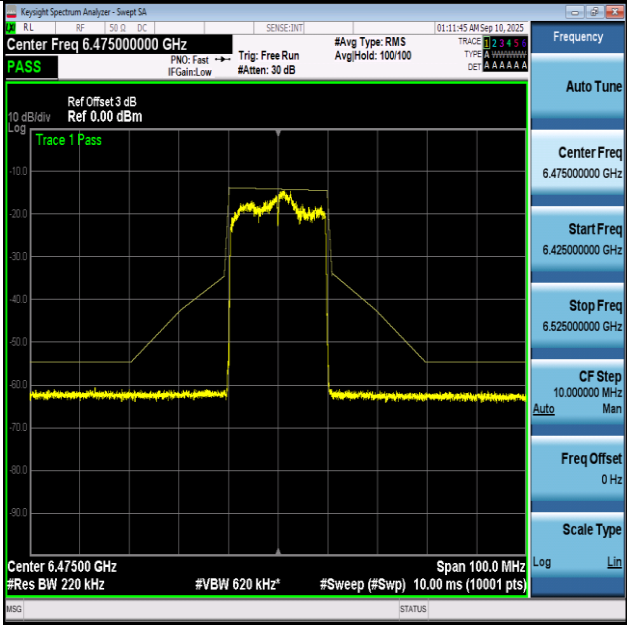
NTNV-11BE20-Ant1+2-6475-PASS
