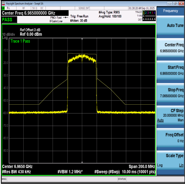
NTNV-11BE40-Ant1+2-6965-PASS
