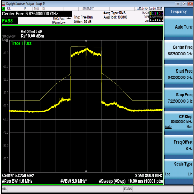
NTNV-11BE160-Ant1+2-6825-PASS
