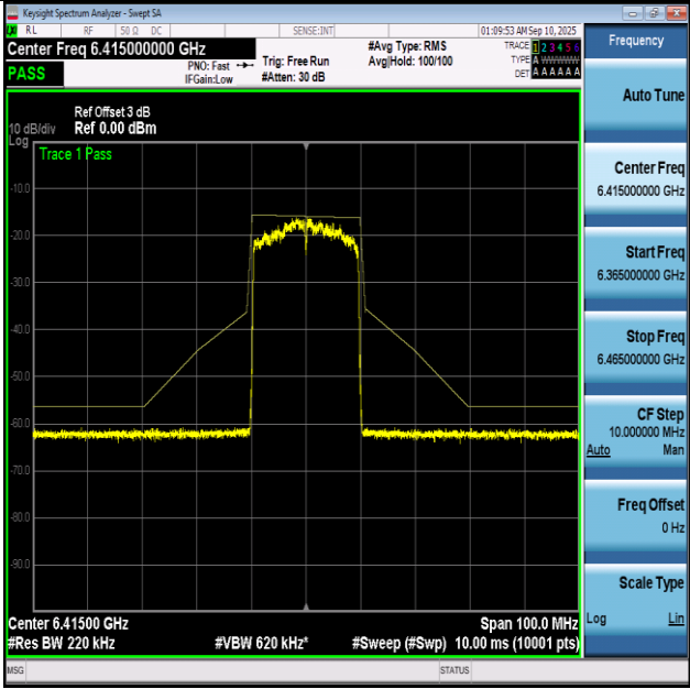
NTNV-11BE20-Ant1+2-6415-PASS
