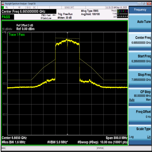
NTNV-11BE160-Ant1+2-6665-PASS
