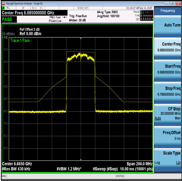
NTNV-11BE40-Ant1+2-6685-PASS
