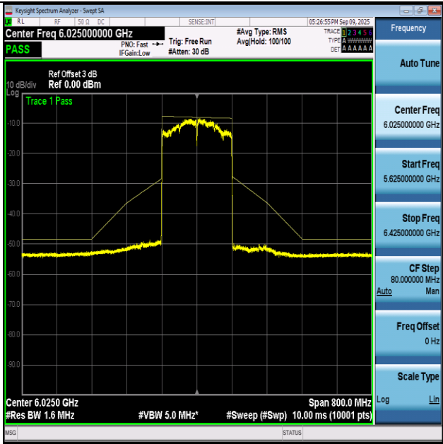
NTNV-11AX160-Ant1+2-6025-PASS
