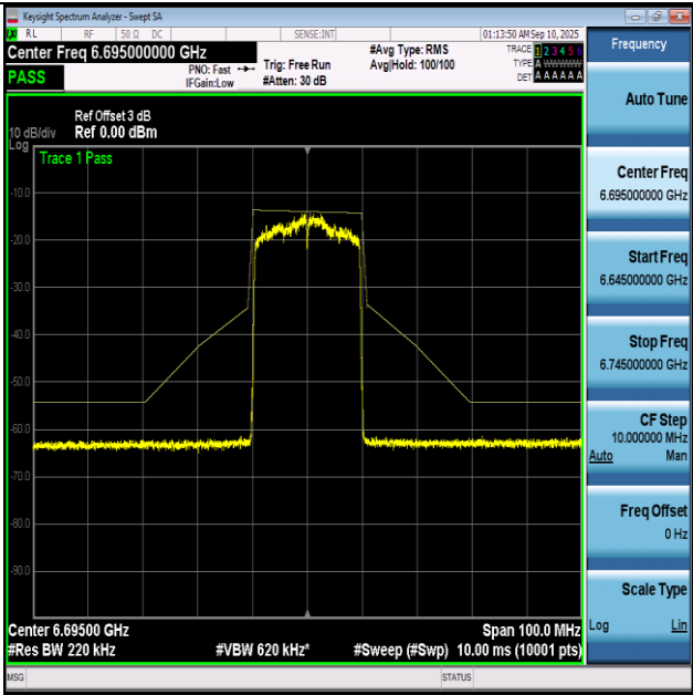
NTNV-11BE20-Ant1+2-6695-PASS
