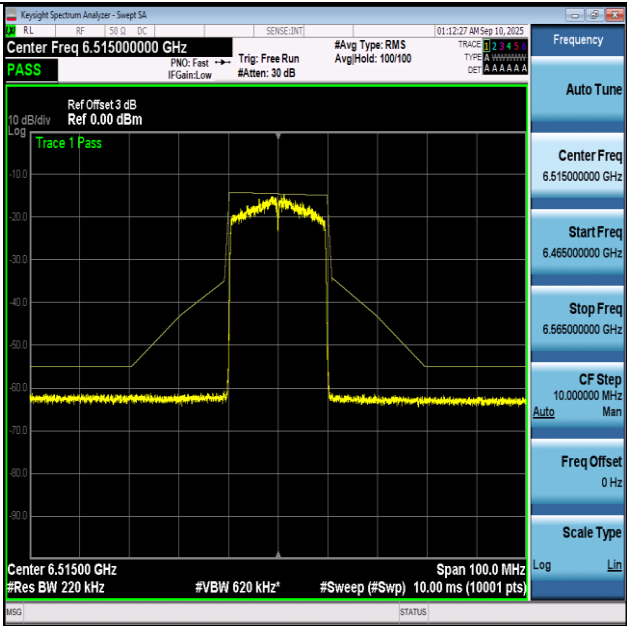
NTNV-11BE20-Ant1+2-6515-PASS
