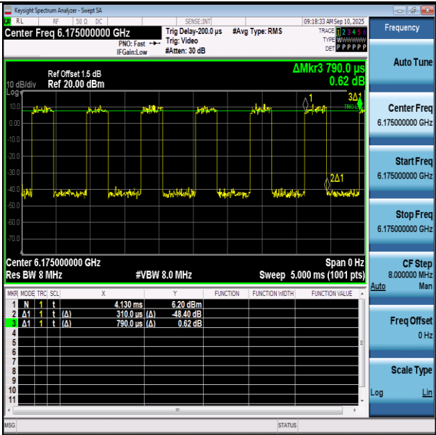
NTNV-11BE20SISO-Ant1-6175
