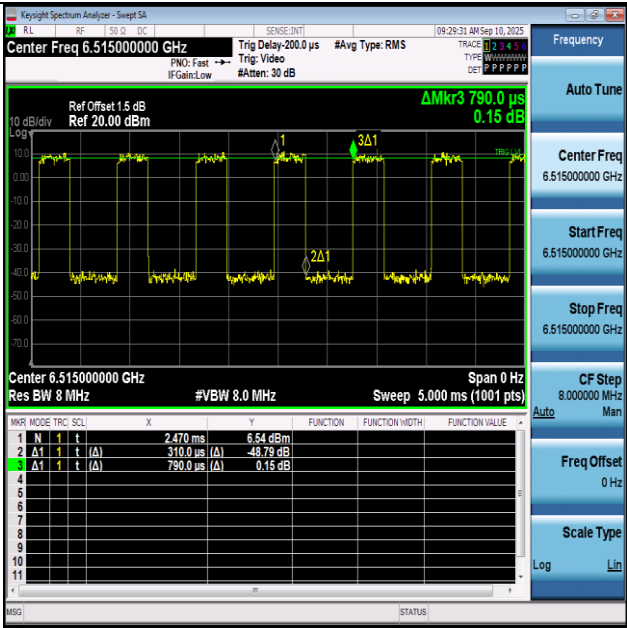
NTNV-11BE20SISO-Ant1-6515
