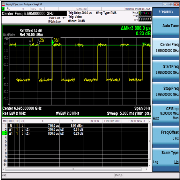
NTNV-11BE20SISO-Ant1-6695
