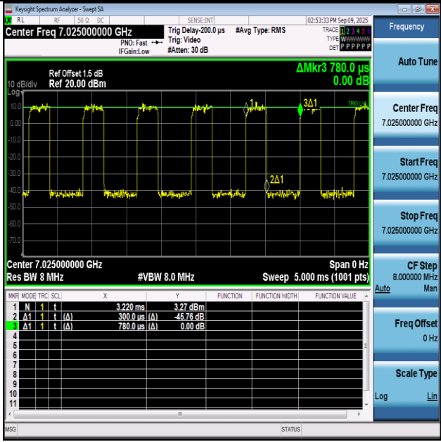
NTNV-11AX80SISO-Ant1-7025
