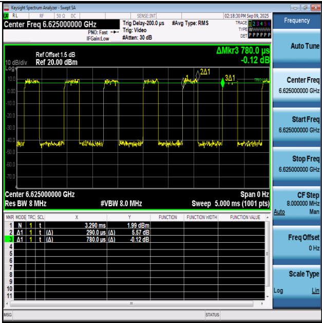
NTNV-11AX80SISO-Ant1-6625
