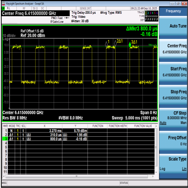
NTNV-11BE20SISO-Ant1-6415
