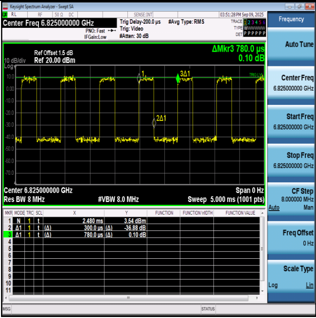
NTNV-11AX160SISO-Ant1-6825
