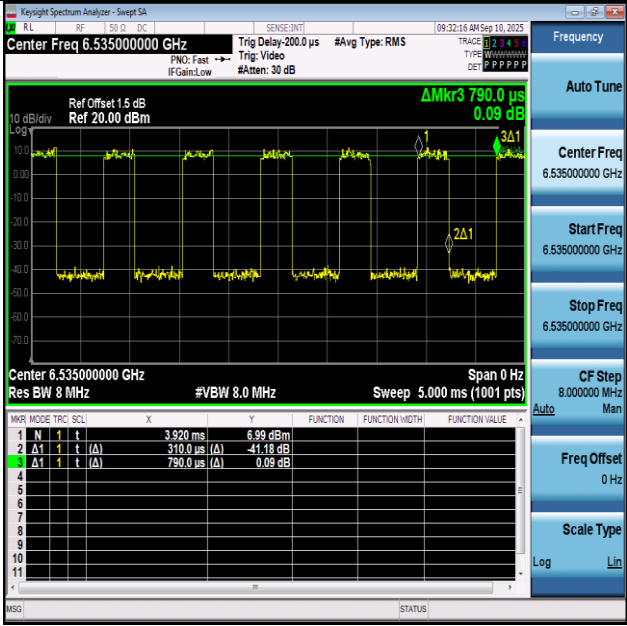
NTNV-11BE20SISO-Ant1-6535
