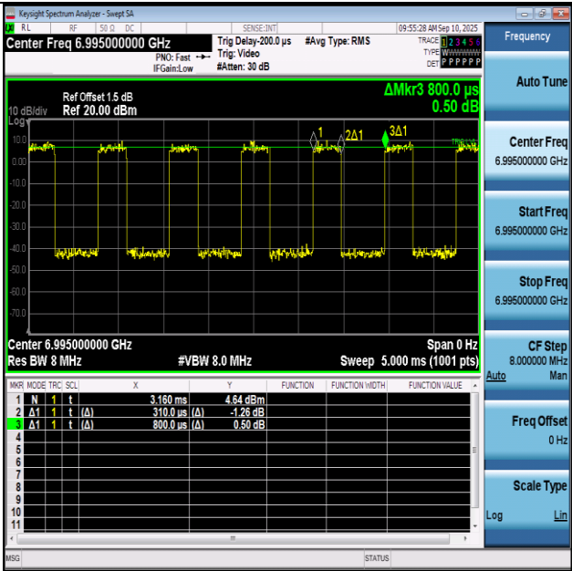
NTNV-11BE20SISO-Ant1-6995
