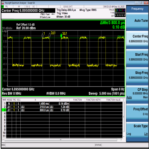
NTNV-11BE20SISO-Ant1-6895
