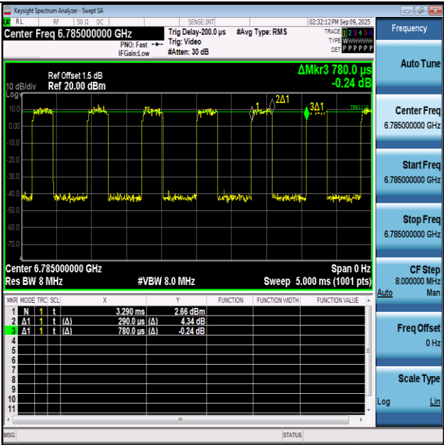
NTNV-11AX80SISO-Ant1-6785
