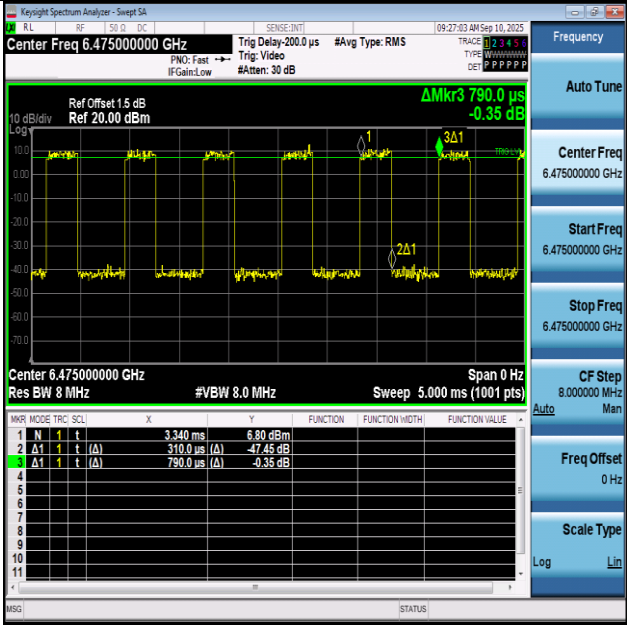
NTNV-11BE20SISO-Ant1-6475
