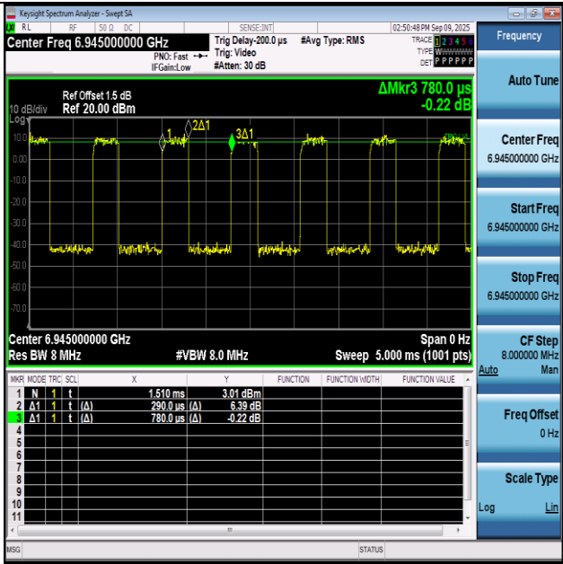
NTNV-11AX80SISO-Ant1-6945
