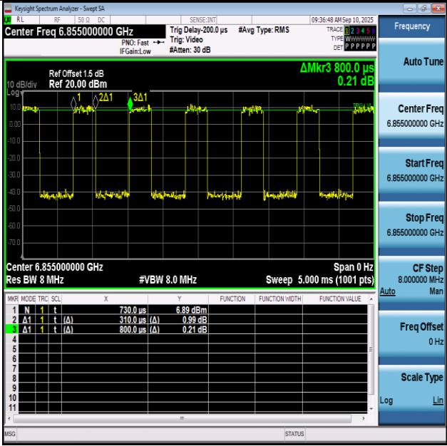
NTNV-11BE20SISO-Ant1-6855
