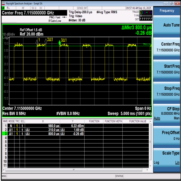
NTNV-11BE20SISO-Ant1-7115
