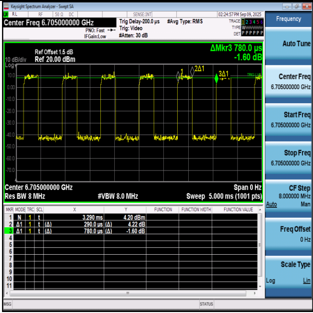
NTNV-11AX80SISO-Ant1-6705
