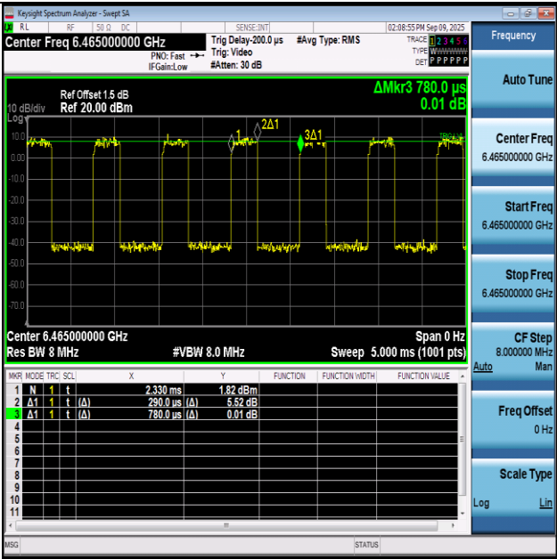
NTNV-11AX80SISO-Ant1-6465
