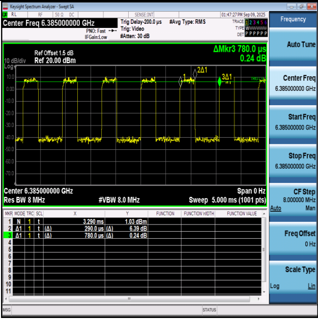
NTNV-11AX80SISO-Ant1-6385
