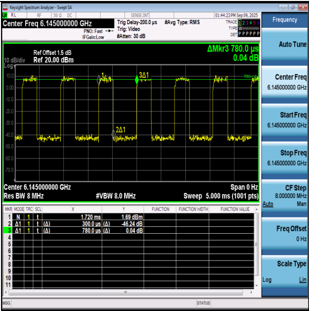
NTNV-11AX80SISO-Ant1-6145
