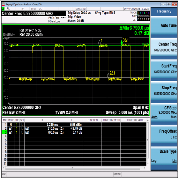
NTNV-11BE20SISO-Ant1-6875
