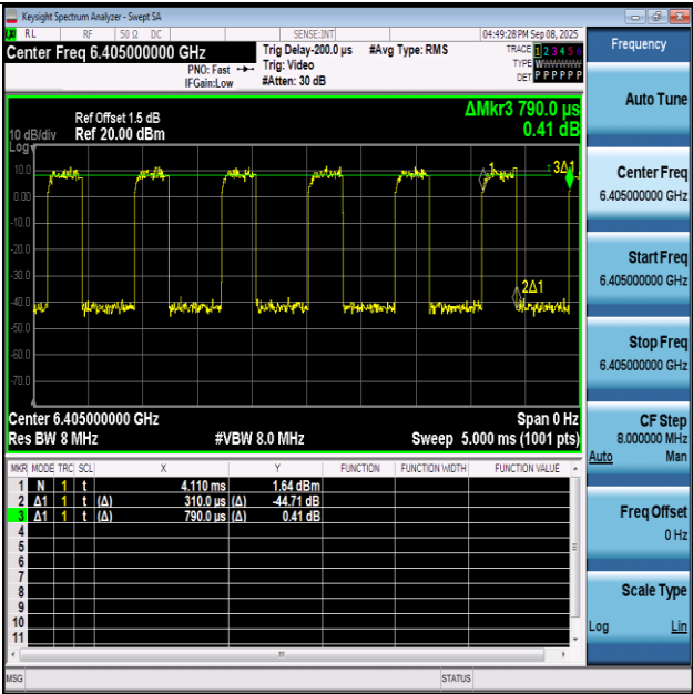
NTNV-11AX40SISO-Ant1-6405
