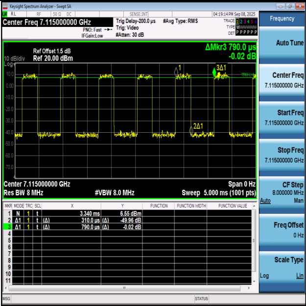
NTNV-11AX20SISO-Ant1-7115
