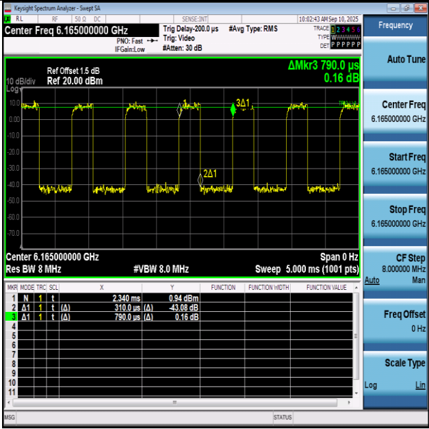
NTNV-11BE40SISO-Ant1-6165
