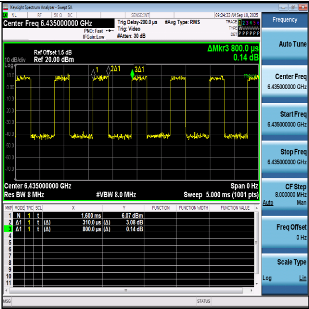
NTNV-11BE20SISO-Ant1-6435
