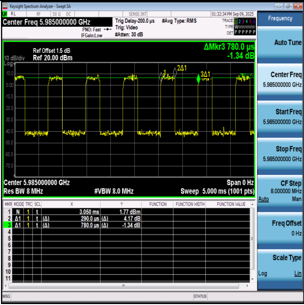
NTNV-11AX80SISO-Ant1-5985
