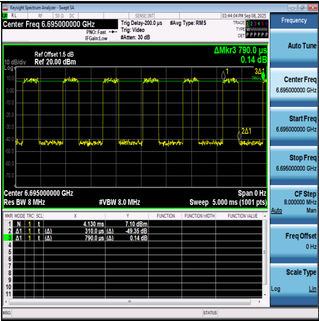
NTNV-11AX20SISO-Ant1-6695
