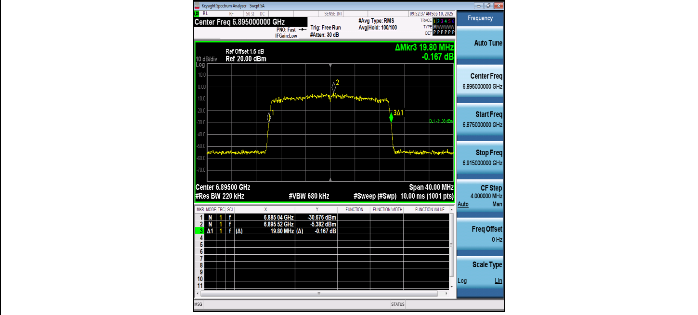
11BE20SISO-Ant1-6895
