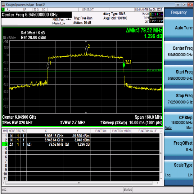
11AX80SISO-Ant1-6945
