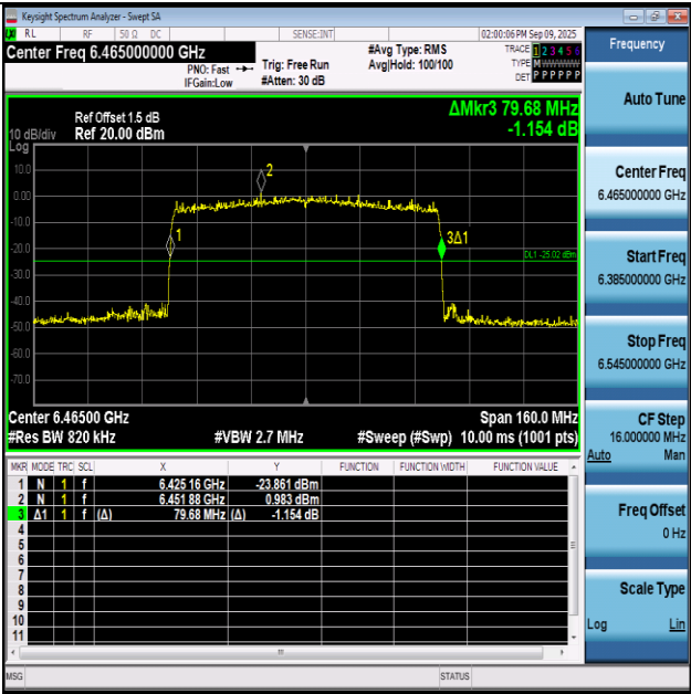
11AX80SISO-Ant1-6465
