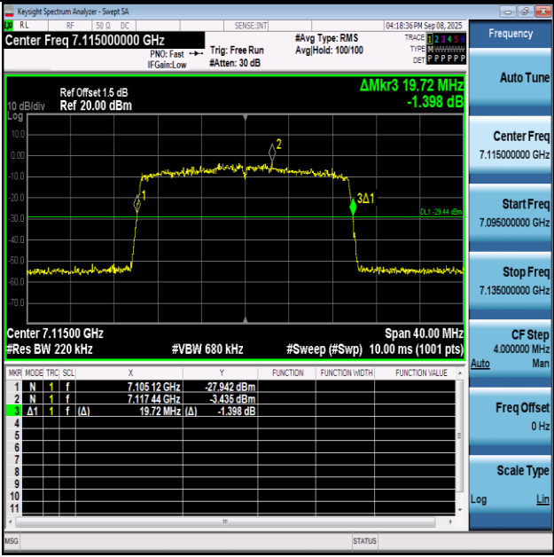
11AX20SISO-Ant1-7115
