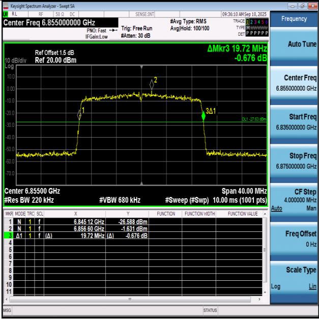
11BE20SISO-Ant1-6855
