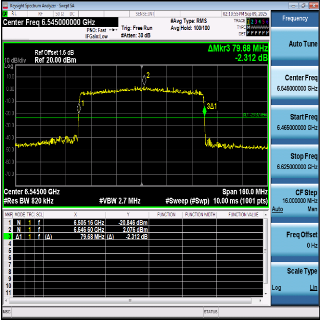
11AX80SISO-Ant1-6545
