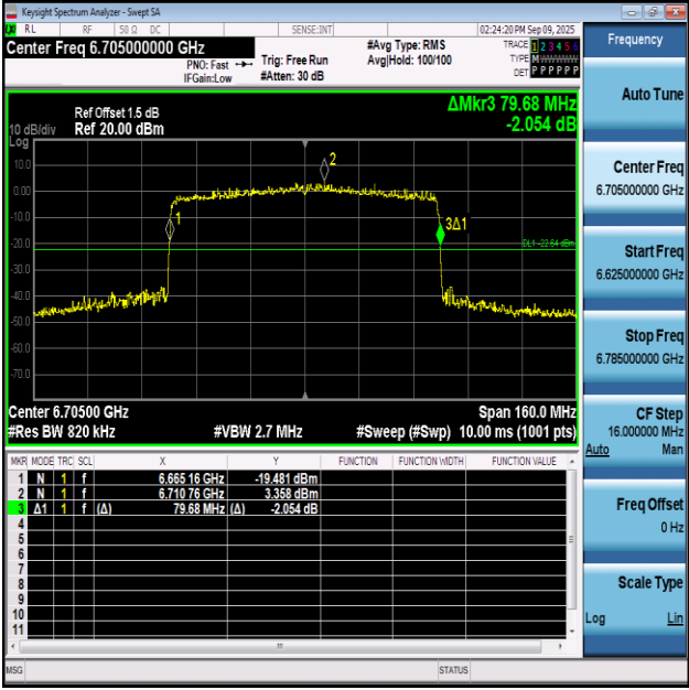
11AX80SISO-Ant1-6705
