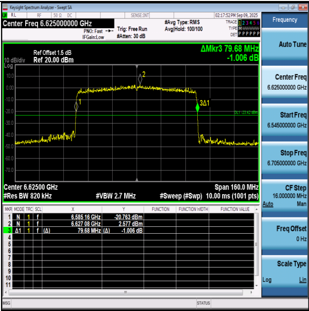
11AX80SISO-Ant1-6625
