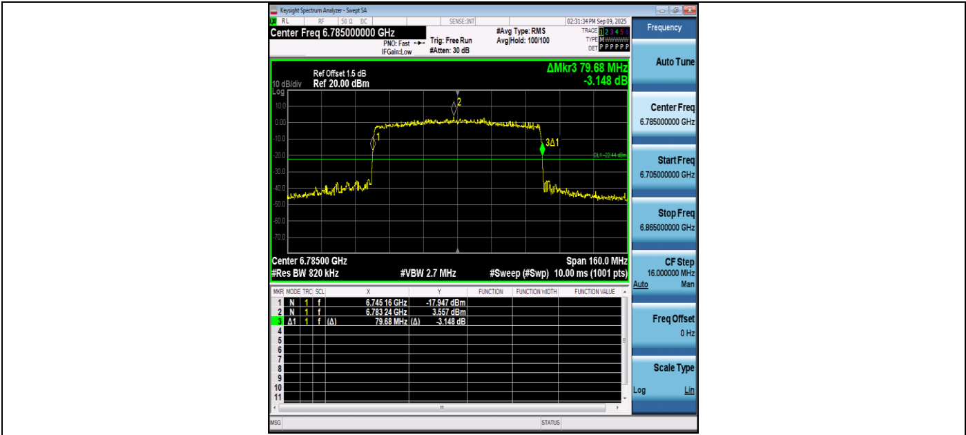
11AX80SISO-Ant1-6785
