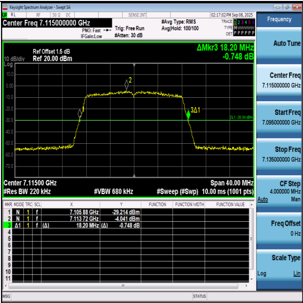
11A-Ant1-7115
