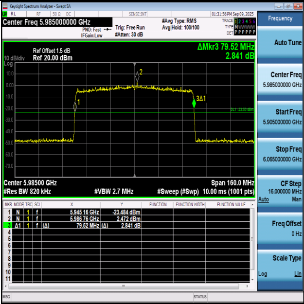
11AX80SISO-Ant1-5985
