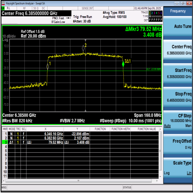
11AX80SISO-Ant1-6385
