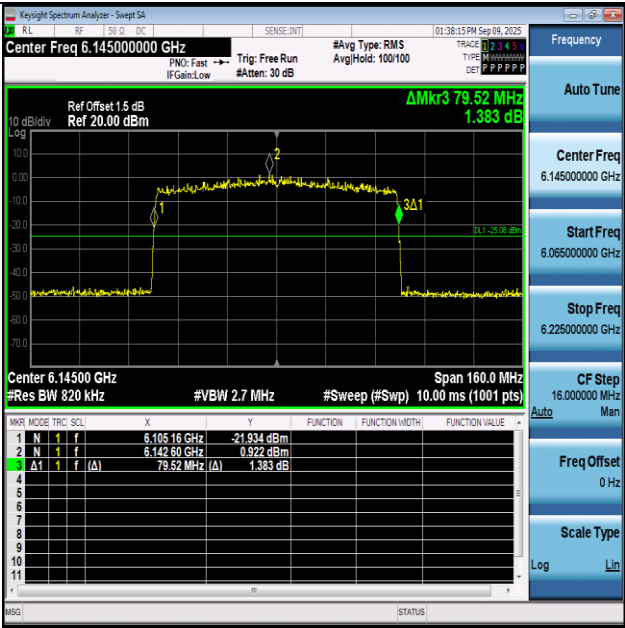
11AX80SISO-Ant1-6145
