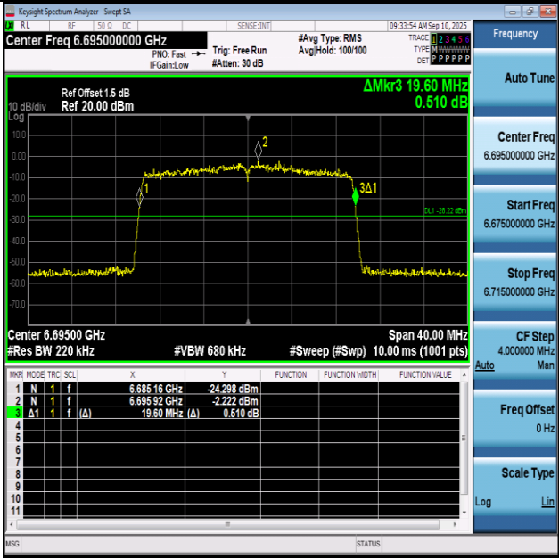
11BE20SISO-Ant1-6695
