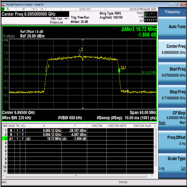
11AX20SISO-Ant1-6695
