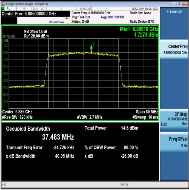
11AX40SISO-Ant1-6885-PASS
