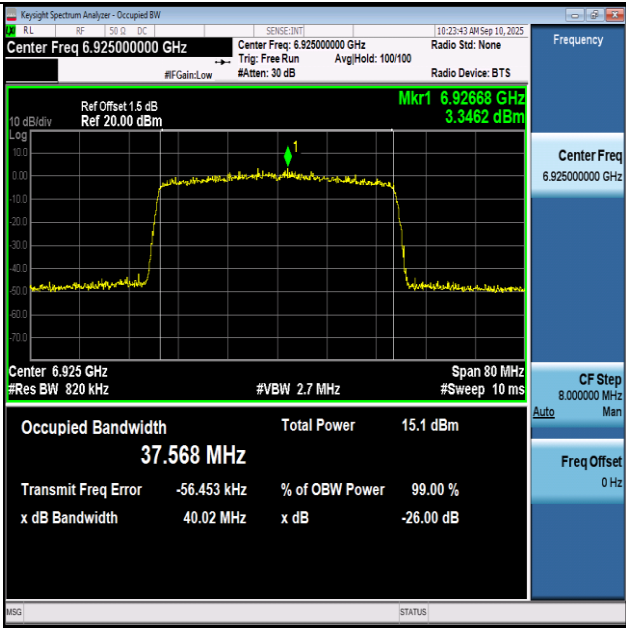
11BE40SISO-Ant1-6925-PASS
