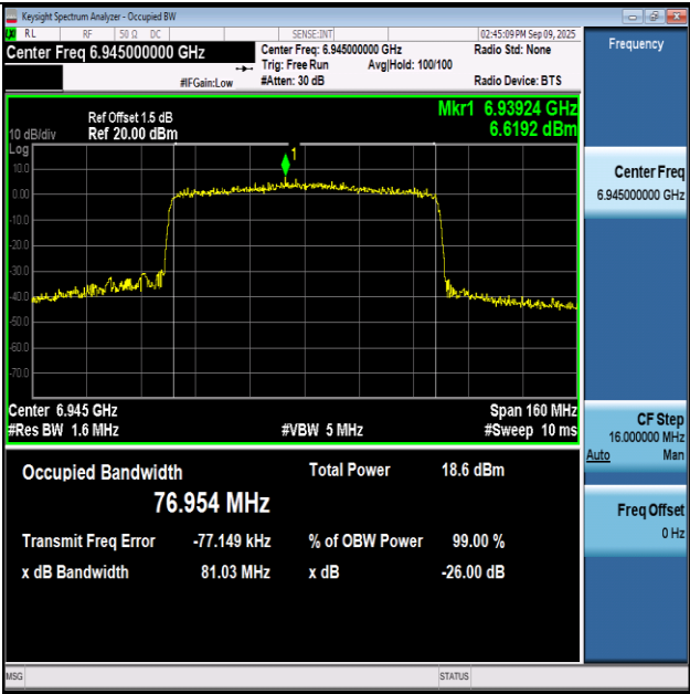
11AX80SISO-Ant1-6945-PASS
