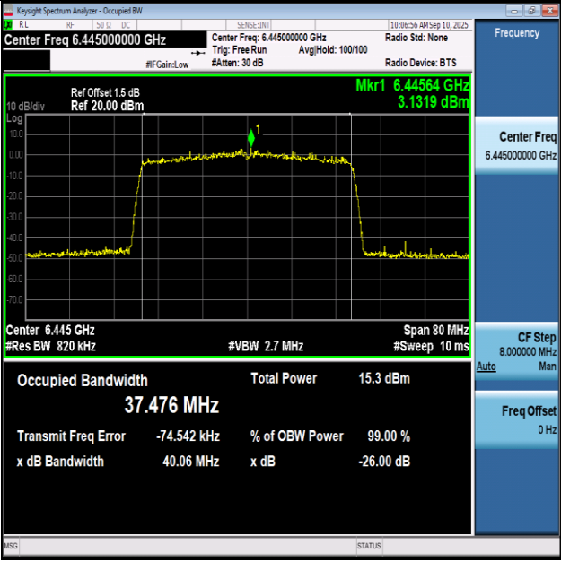
11BE40SISO-Ant1-6445-PASS
