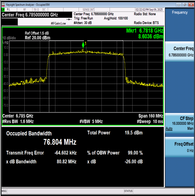
11AX80SISO-Ant1-6785-PASS
