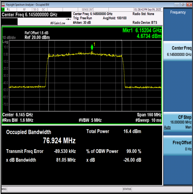
11AX80SISO-Ant1-6145-PASS
