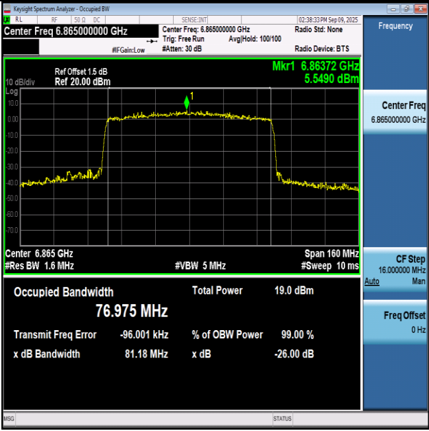
11AX80SISO-Ant1-6865-PASS
