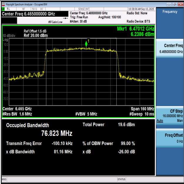
11BE80SISO-Ant1-6465-PASS
