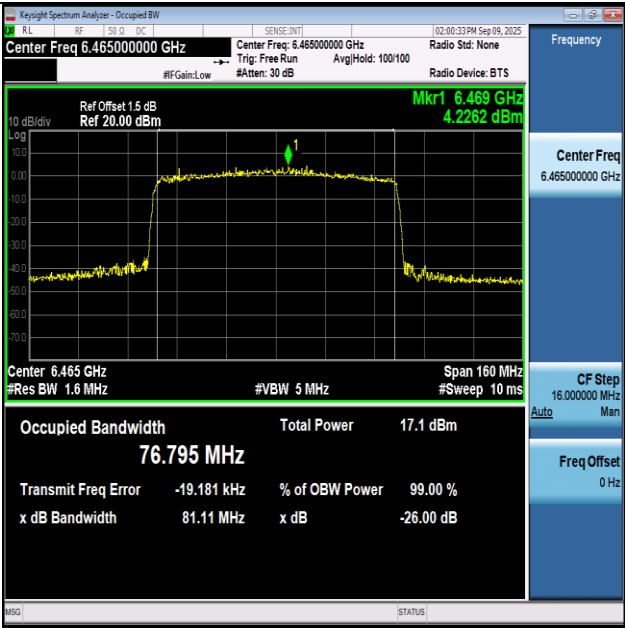
11AX80SISO-Ant1-6465-PASS
