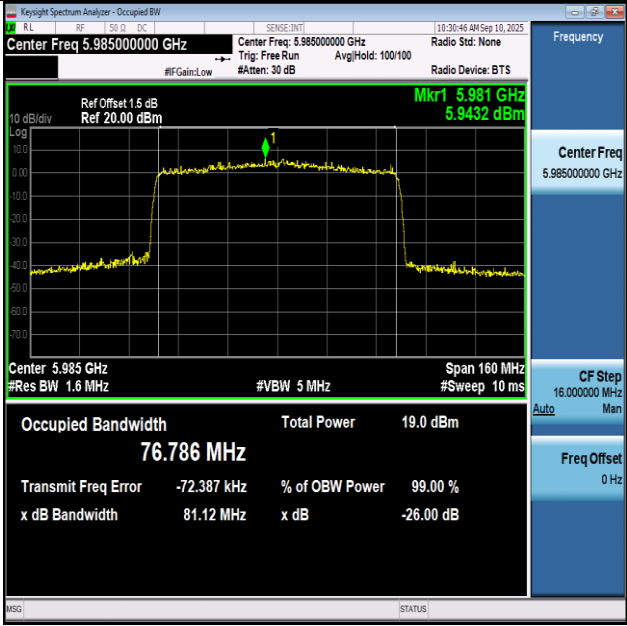
11BE80SISO-Ant1-5985-PASS
