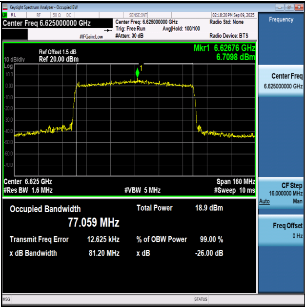
11AX80SISO-Ant1-6625-PASS
