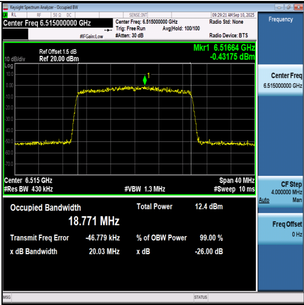
11BE20SISO-Ant1-6515-PASS
