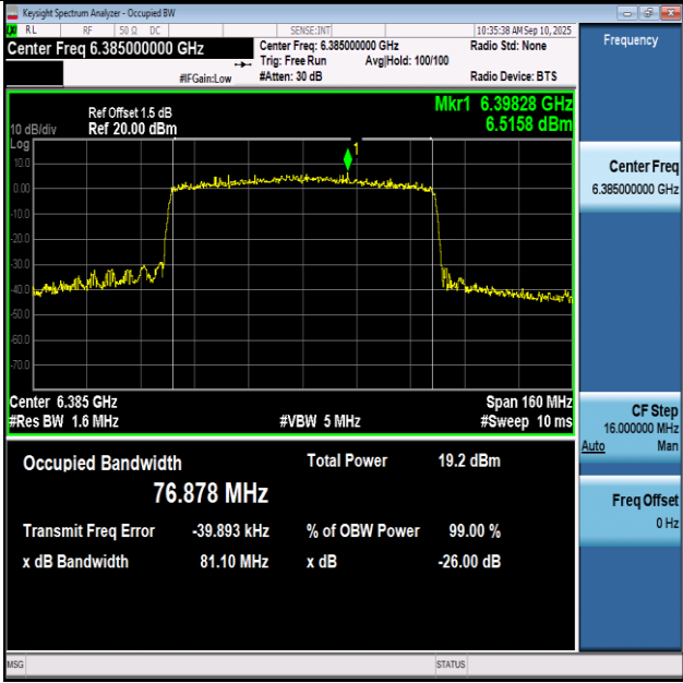
11BE80SISO-Ant1-6385-PASS
