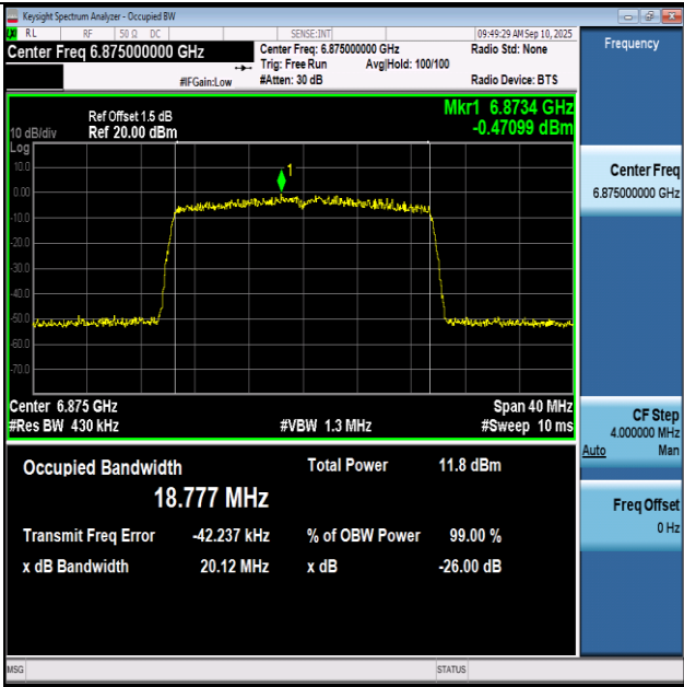
11BE20SISO-Ant1-6875-PASS
