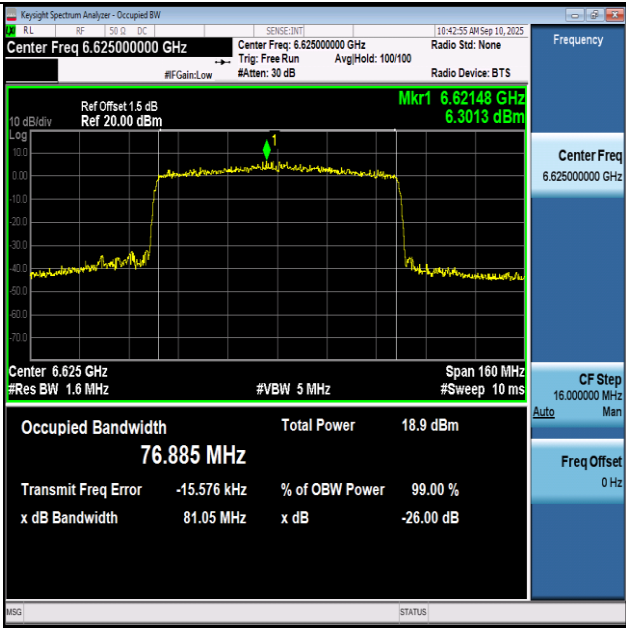
11BE80SISO-Ant1-6625-PASS
