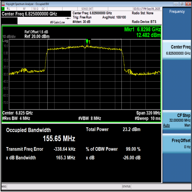
11AX160SISO-Ant1-6825-PASS
