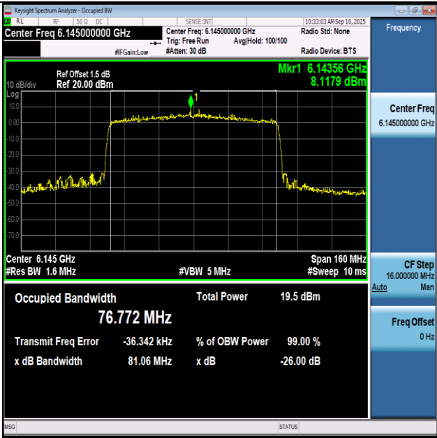
11BE80SISO-Ant1-6145-PASS
