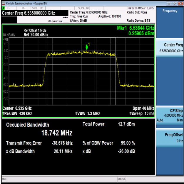
11BE20SISO-Ant1-6535-PASS
