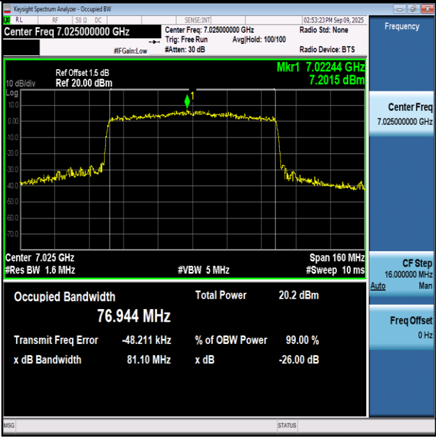
11AX80SISO-Ant1-7025-PASS
