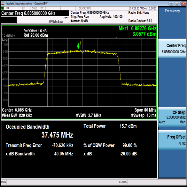
11BE40SISO-Ant1-6885-PASS
