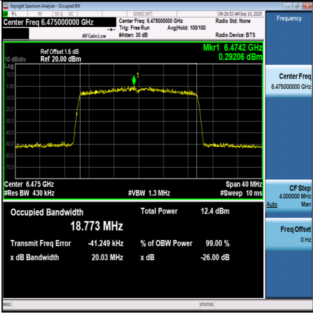
11BE20SISO-Ant1-6475-PASS
