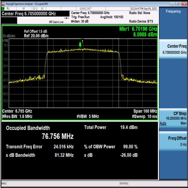
11AX80SISO-Ant1-6705-PASS
