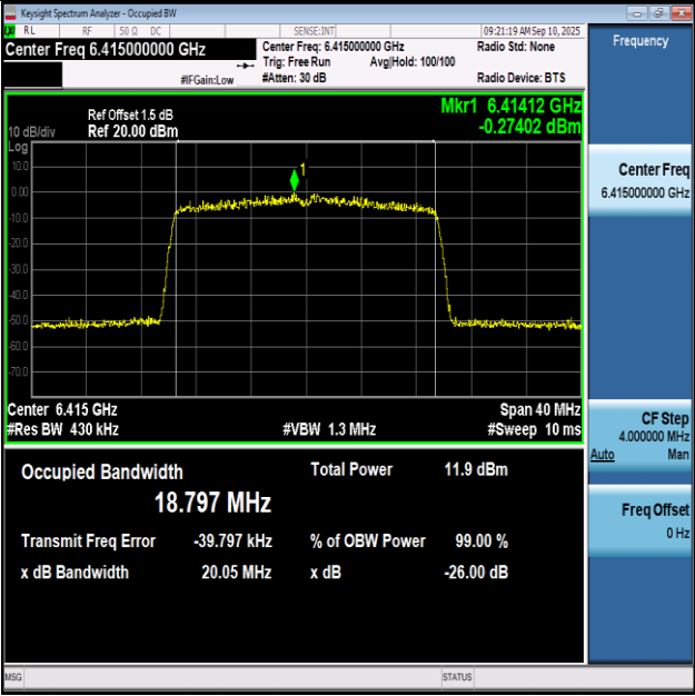
11BE20SISO-Ant1-6415-PASS
