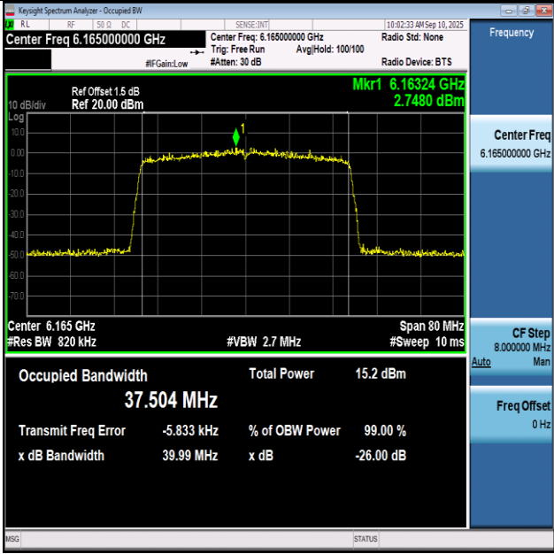
11BE40SISO-Ant1-6165-PASS
