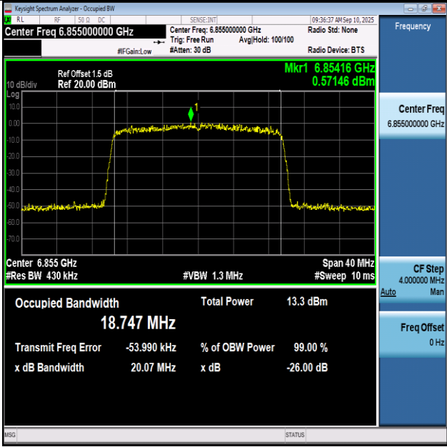
11BE20SISO-Ant1-6855-PASS
