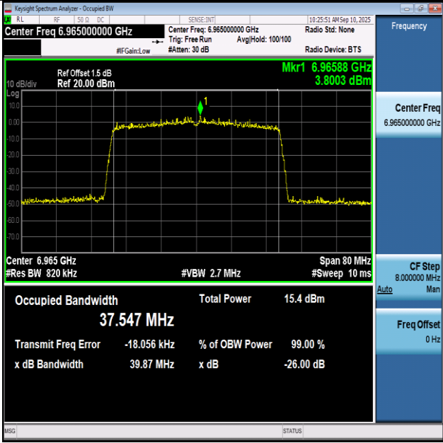
11BE40SISO-Ant1-6965-PASS
