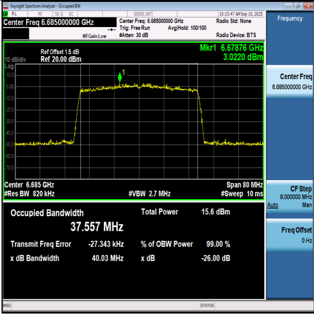
11BE40SISO-Ant1-6685-PASS
