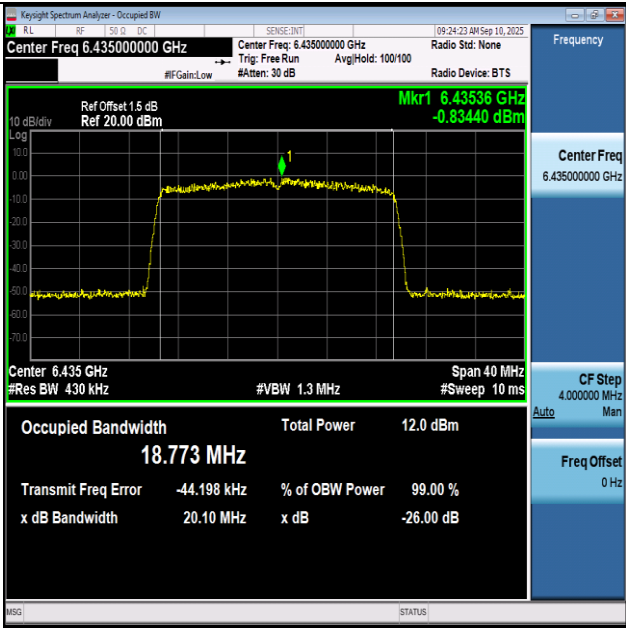
11BE20SISO-Ant1-6435-PASS
