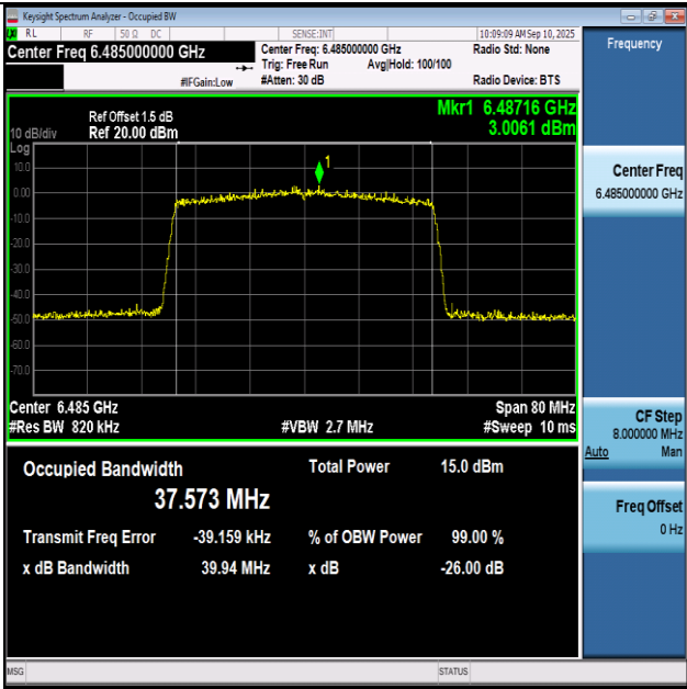
11BE40SISO-Ant1-6485-PASS
