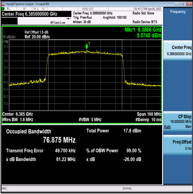
11AX80SISO-Ant1-6385-PASS
