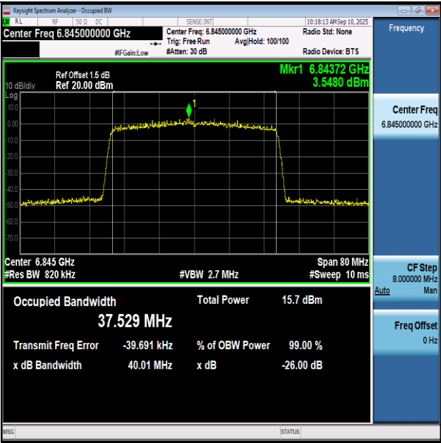
11BE40SISO-Ant1-6845-PASS
