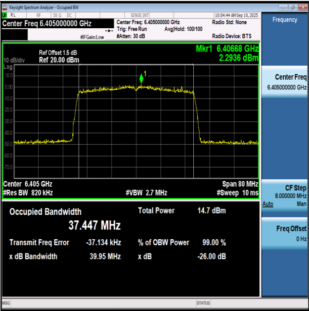
11BE40SISO-Ant1-6405-PASS
