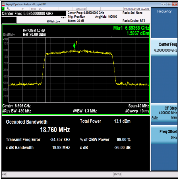
11BE20SISO-Ant1-6695-PASS
