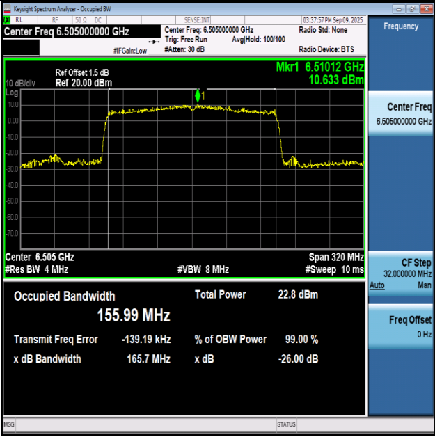
11AX160SISO-Ant1-6505-PASS
