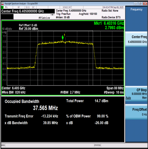
11AX40SISO-Ant1-6405-PASS
