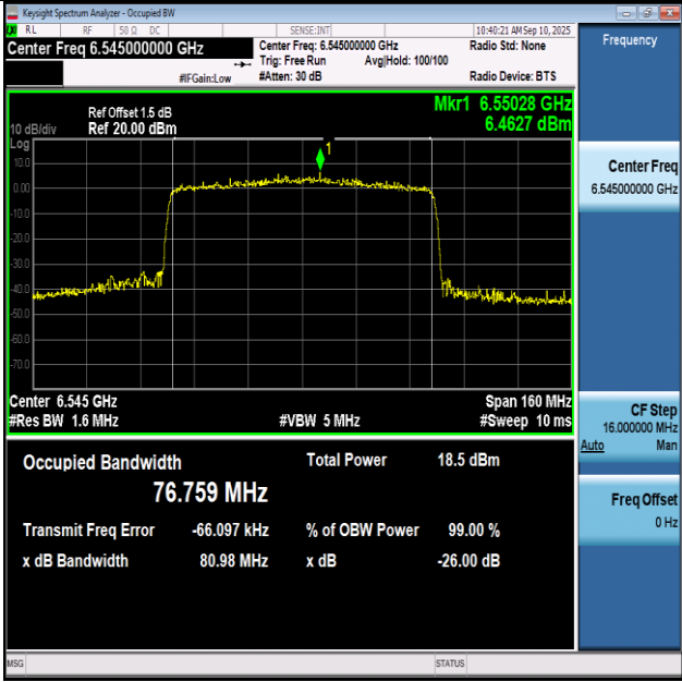
11BE80SISO-Ant1-6545-PASS
