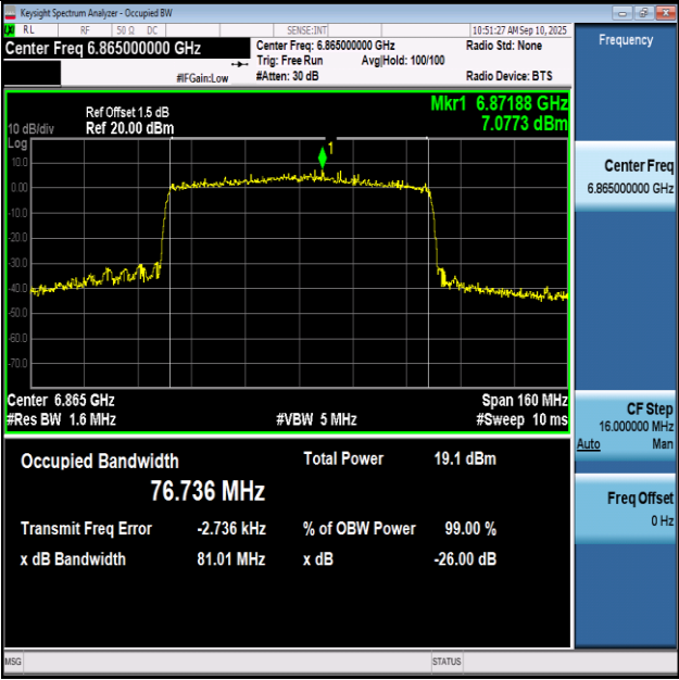
11BE80SISO-Ant1-6865-PASS
