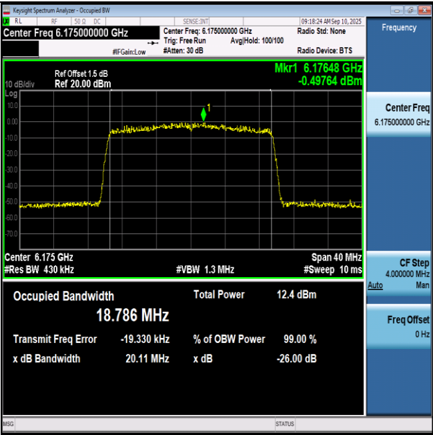
11BE20SISO-Ant1-6175-PASS
