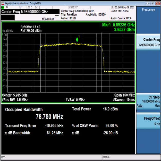
11AX80SISO-Ant1-5985-PASS
