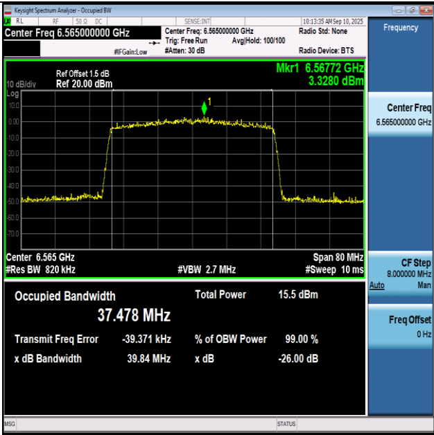
11BE40SISO-Ant1-6565-PASS
