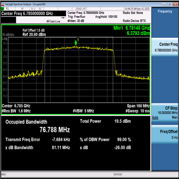
11BE80SISO-Ant1-6785-PASS
