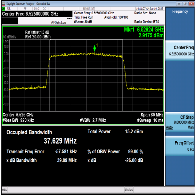
11BE40SISO-Ant1-6525-PASS
