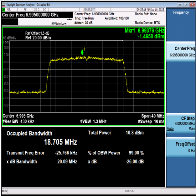
11BE20SISO-Ant1-6995-PASS
