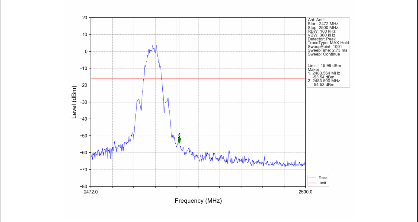
2M_HCH_2480MHz_Ant1_NTNV
