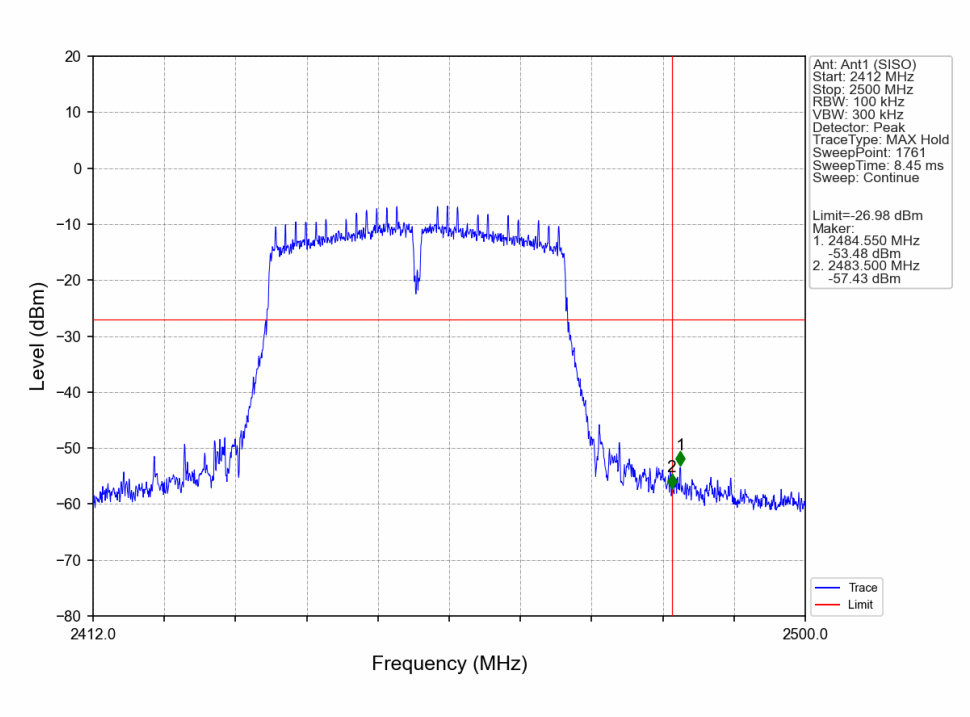
802.11n(HT40)_HCH_2452MHz_Ant1_NTNV
