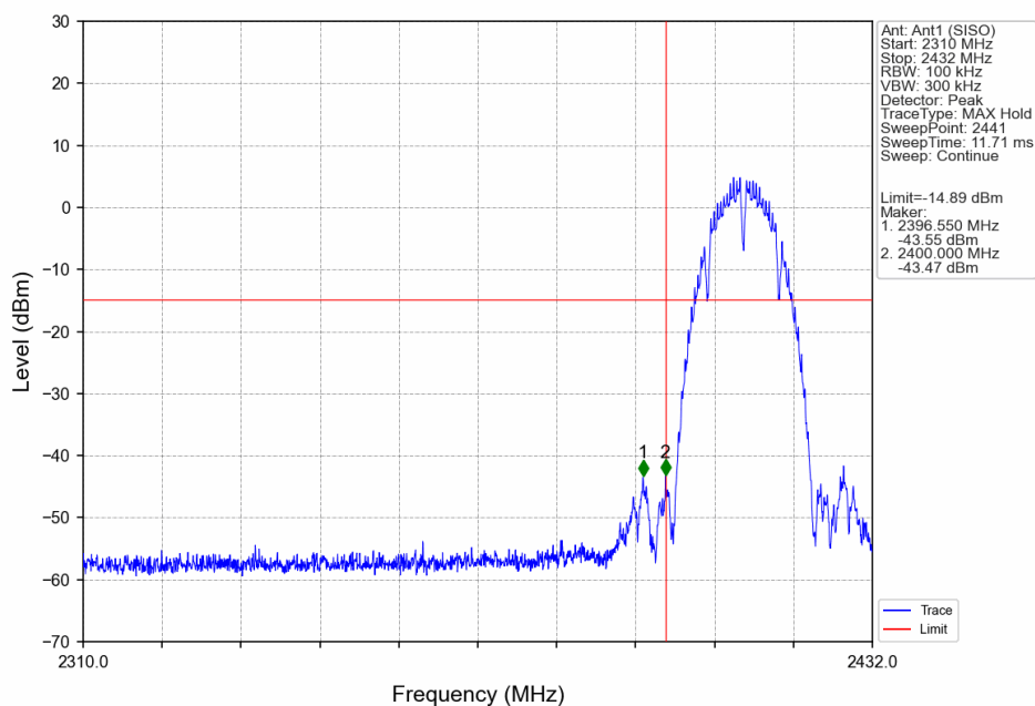
802.11b_LCH_2412MHz_Ant1_NTNV
