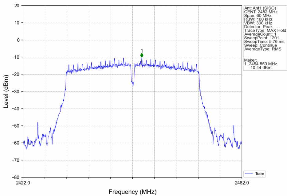
802.11n(HT40)_HCH_2452MHz_Ant1_NTNV
