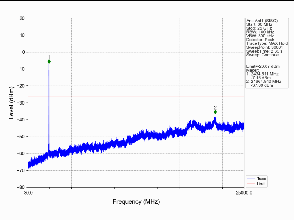
802.11n(HT40)_HCH_2452MHz_Ant1_NTNV
