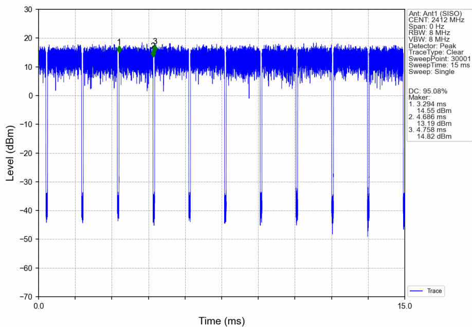
802.11n(HT20)_LCH_2412MHz_Ant1_NTNV
