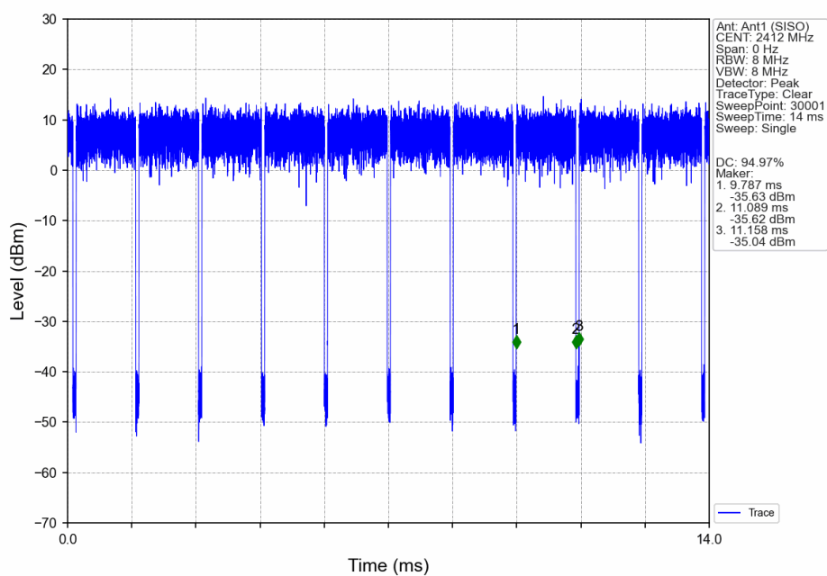
802.11n(HT20)_LCH_2412MHz_Ant1_NTNV
