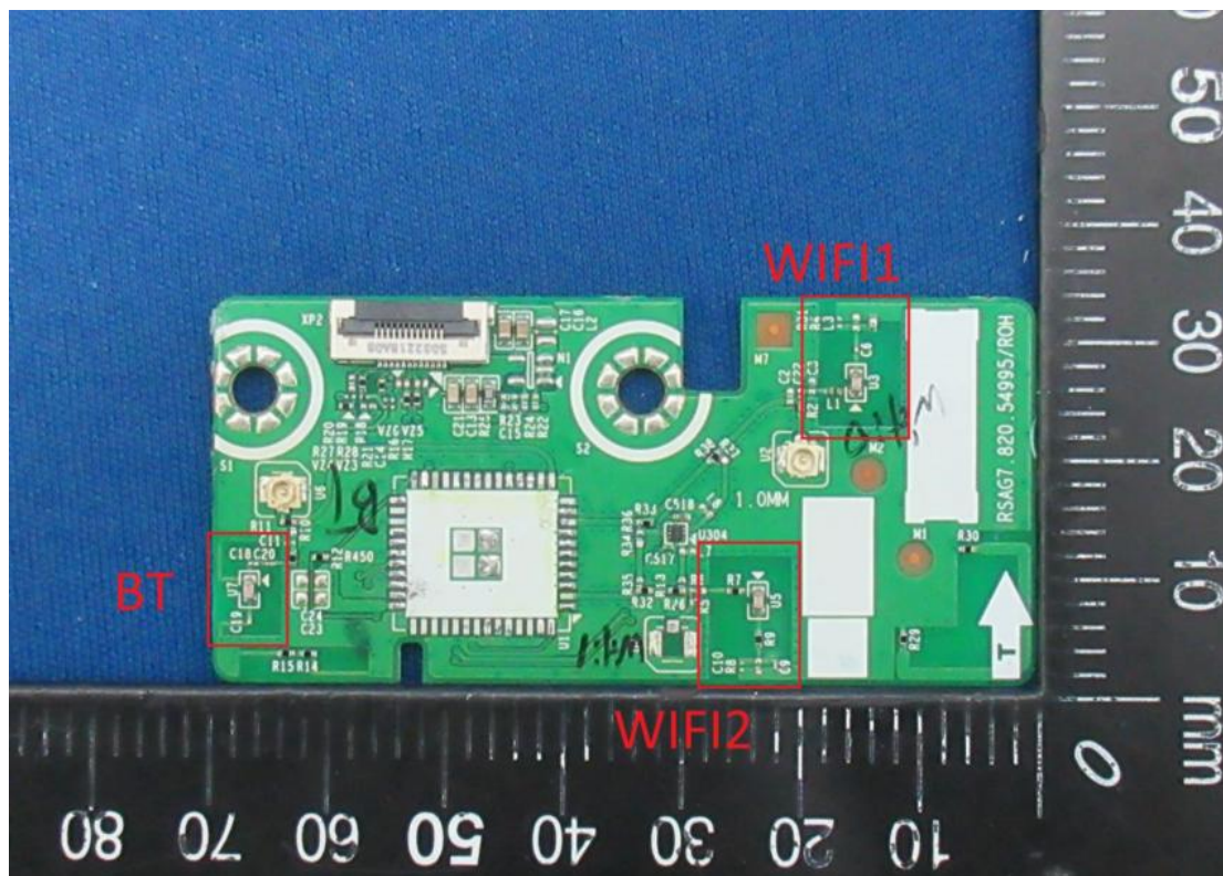
Antenna Set 1
