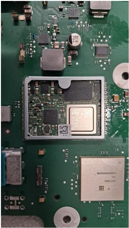
Figure 1.4 Radio module
