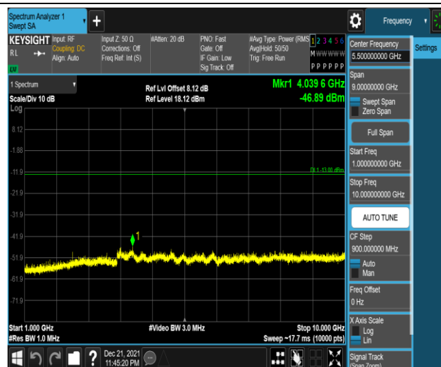
Band13-5MHz-QPSK-23255-1RB#0-Range4:1000~10000MHz
