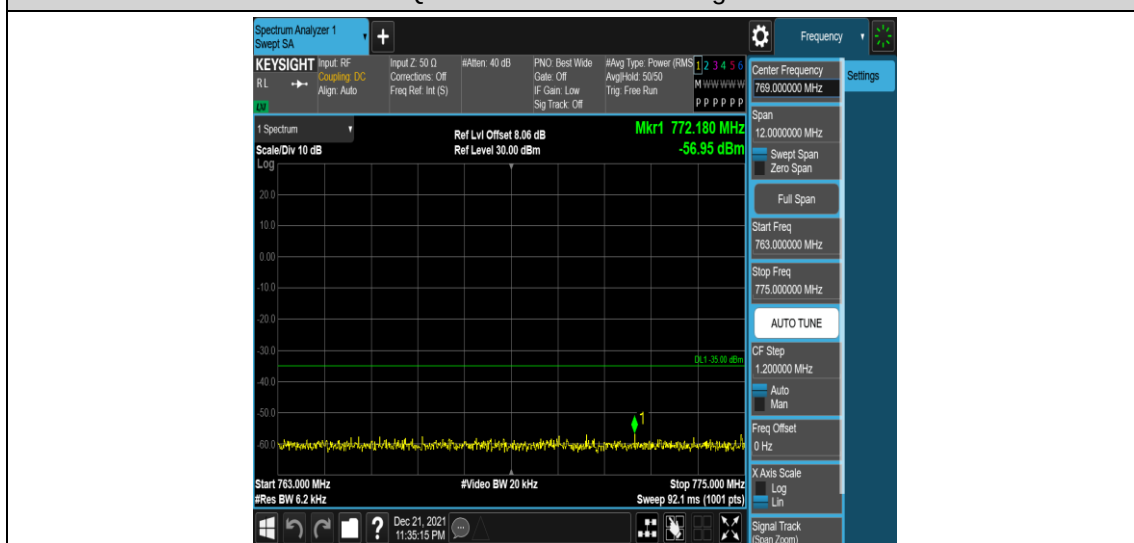
Band13-5MHz-QPSK-23205-1RB#0-Range5:763~775MHz
