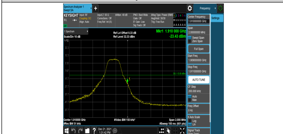
Band2-3MHz-QPSK-19185-1RB#14
