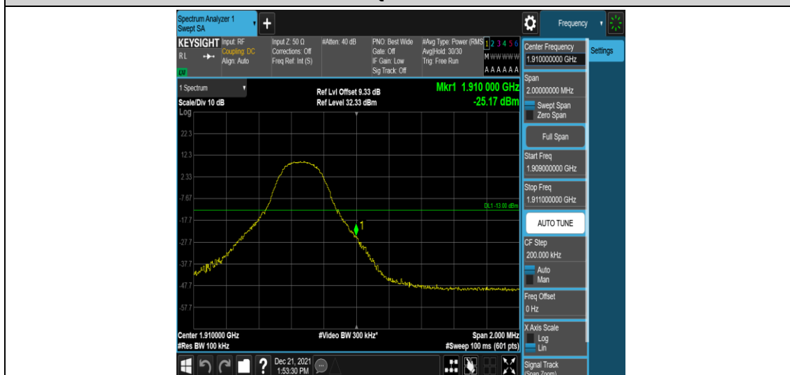
Band2-5MHz-QPSK-19175-1RB#24
