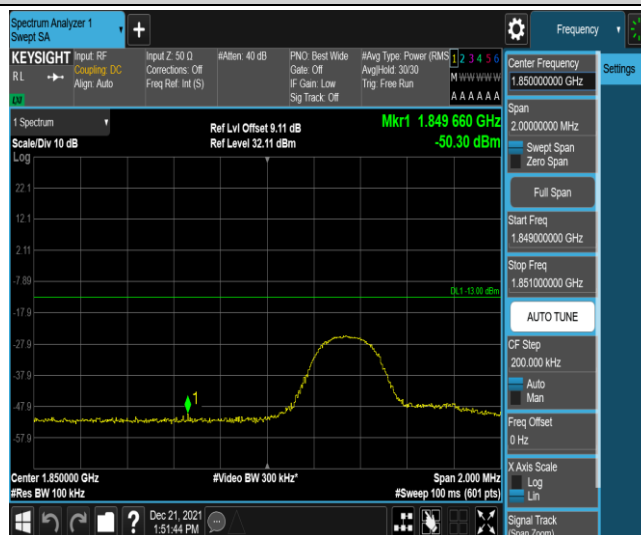
Band2-5MHz-QPSK-18625-1RB#24
